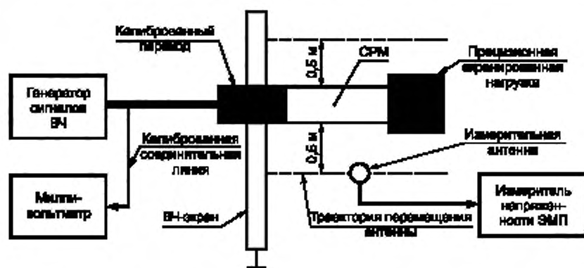
Рисунок 3 — Расположение СРМ, СИ и испытательного оборудования при определении напряженности ЭМП вокруг СРМ
