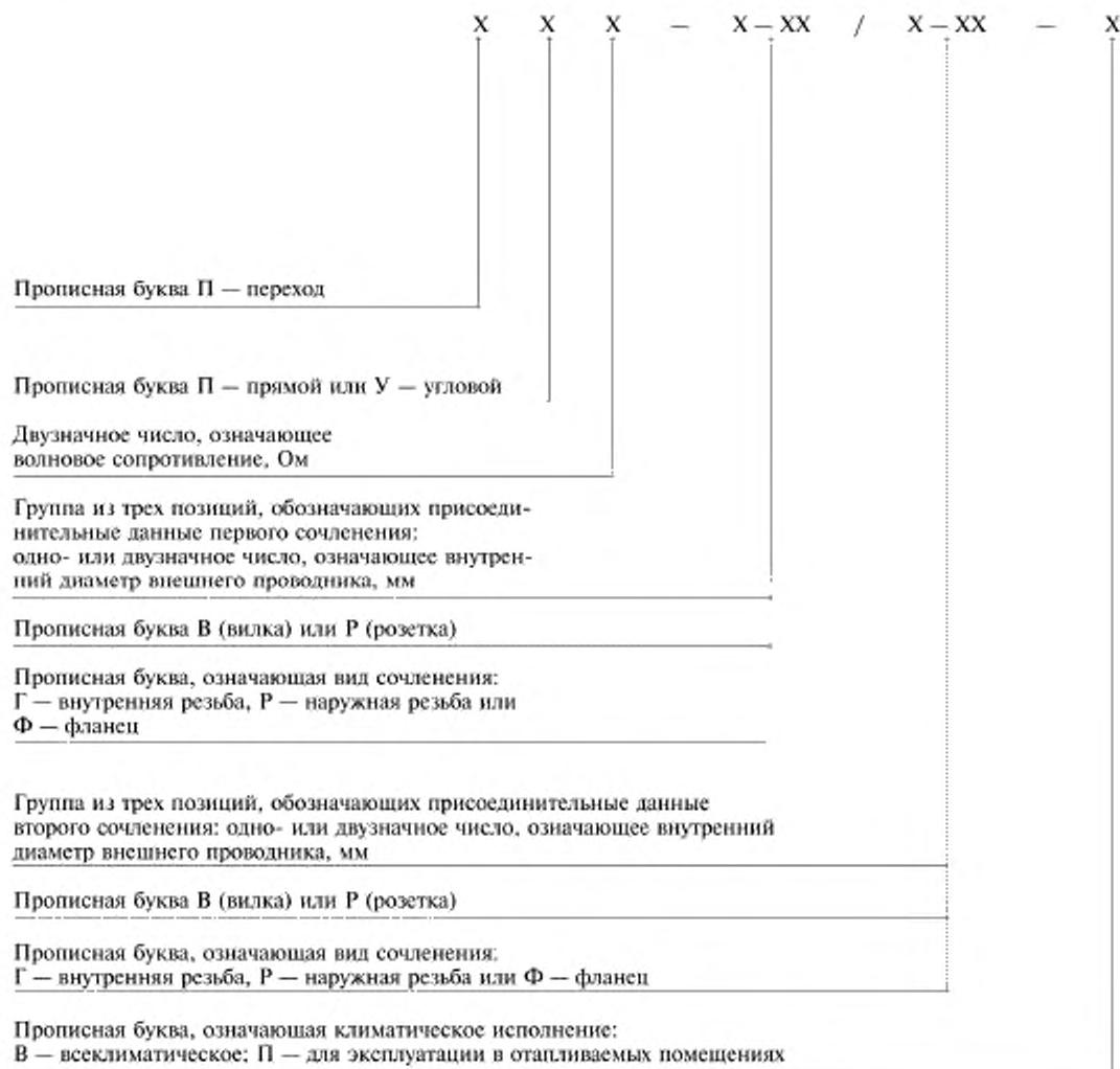
Рисунок 2 — Структура условного обозначения СРМ-перехода
