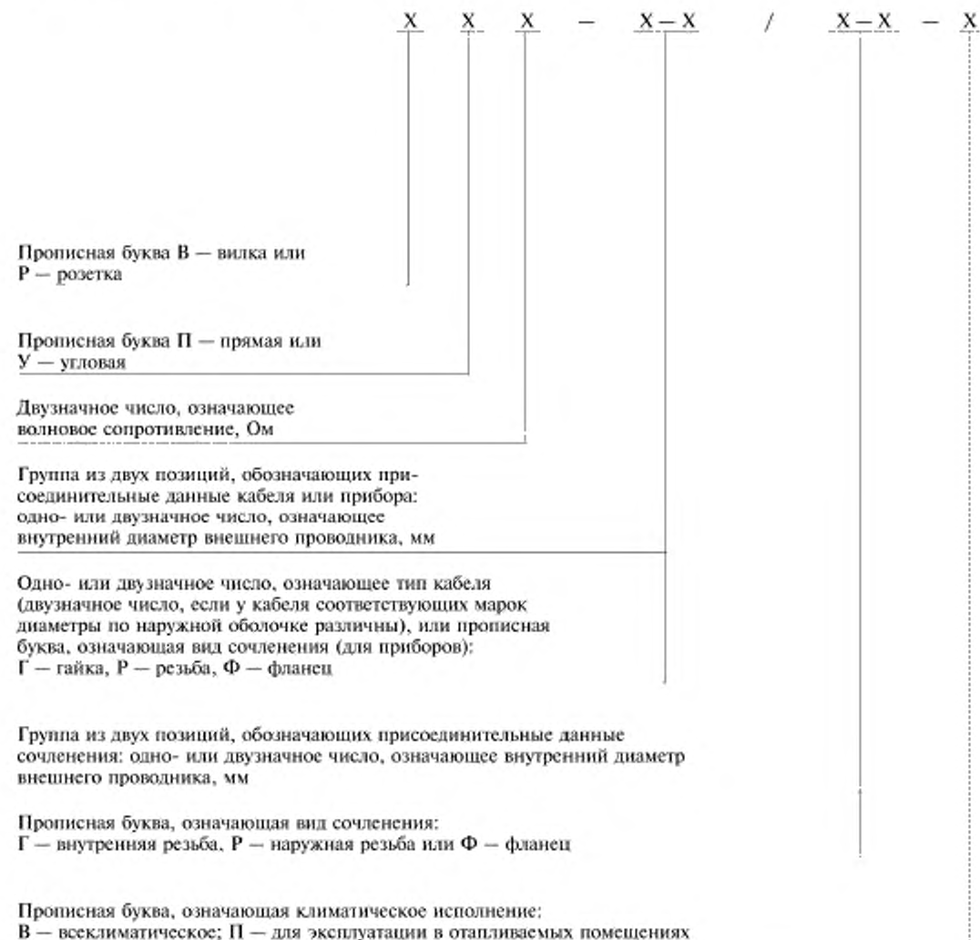
Рисунок 1 — Структура условного обозначения СРМ вилки или розетки
