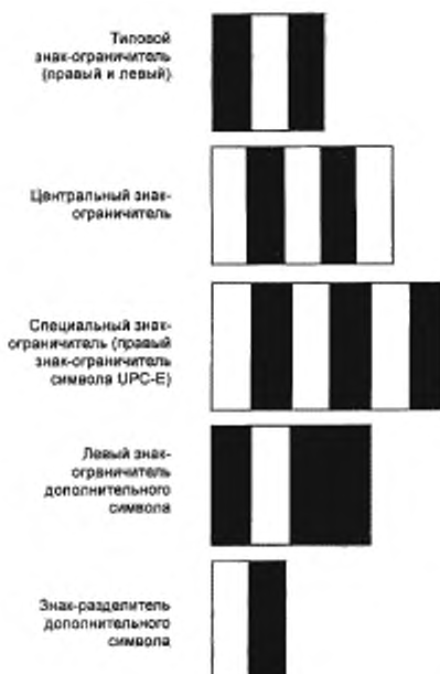
Рисунок D.2 — Представление вспомогательных знаков
