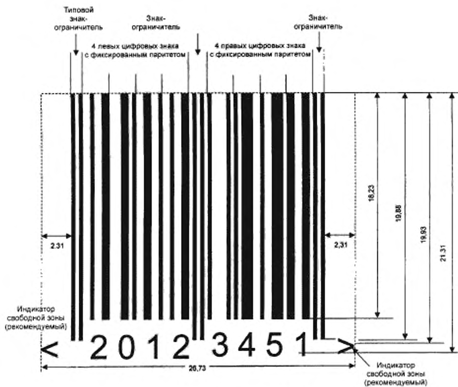
Рисунок Е.4 — Символ EAN-8
