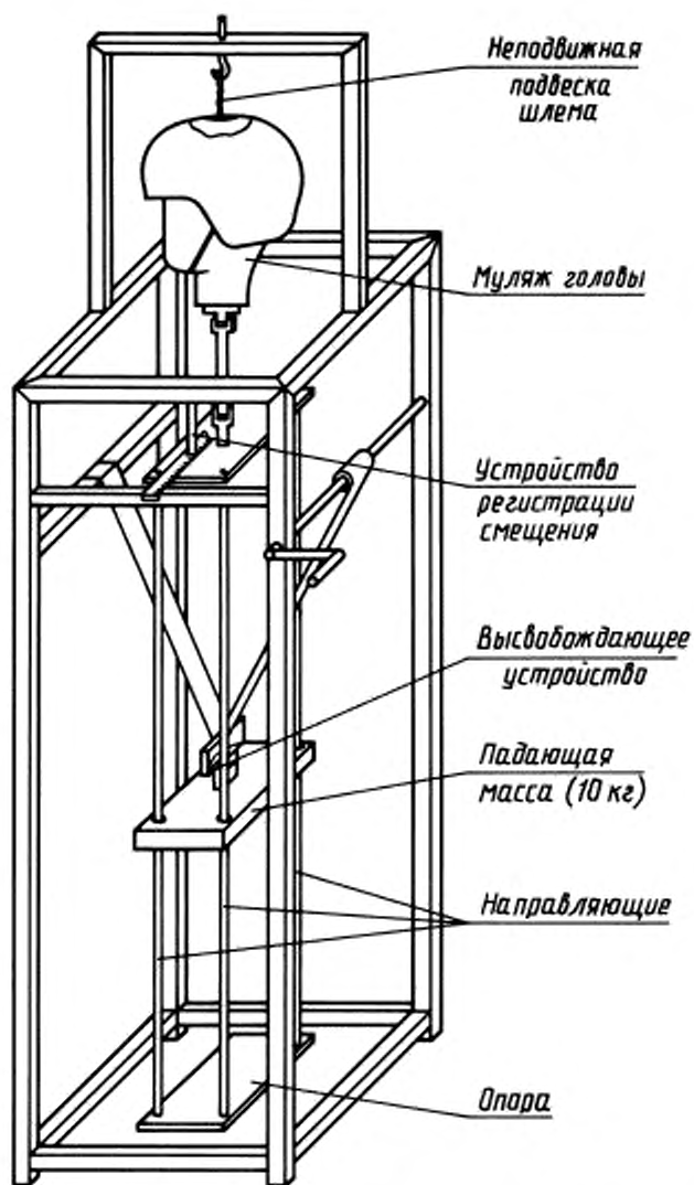
Рисунок 2 — Динамическое испытание удерживающей системы
