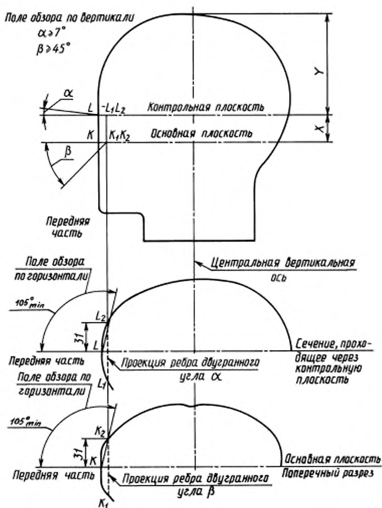
Рисунок 2А — Периферический обзор
