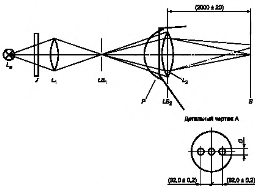
Рисунок 2 — Расположение приспособления для измерения призматической разности
