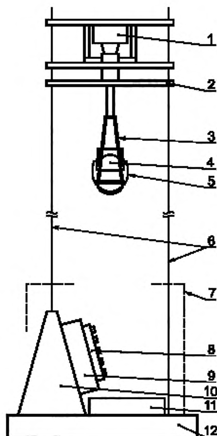
1 — механизм сбрасывания; 2 — тележка; 3 — подвесные ремни; 4 — муфта головы; 5 — шлем; 6 — направляющие тросы; 7 — сетевое ограждение; 8 — опора; 9 — измерительные приборы; 10 — твердый каркас; 11 — подушка, смягчающая удар; 12 — основание
