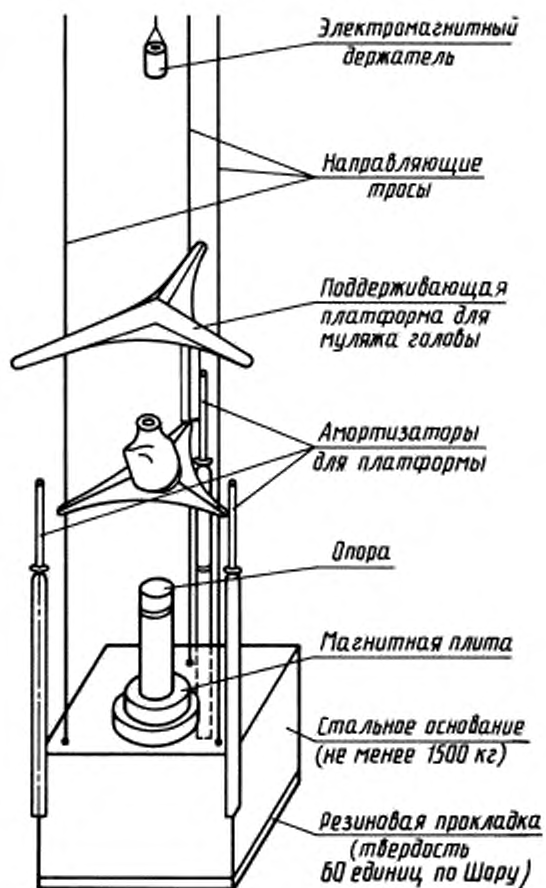
Рисунок 1а — Устройство для сброса муляжа головы
