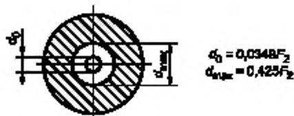
Рисунок 2 — Кольцевая диафрагма D_2
