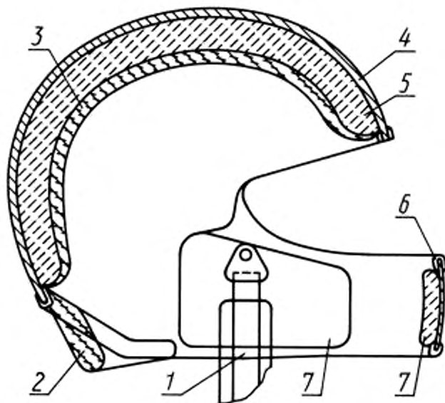
Схема защитного шлема
