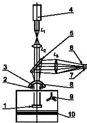
1 — зеркало; 2 — опорное кольцо; 3 — кольцо из мягкой резины; 4 — лазер; 5 — светоделитель; 6 — диафрагма; 7 — приемник; 8 — образец; 9 — вентилятор; 10 — водная баня
