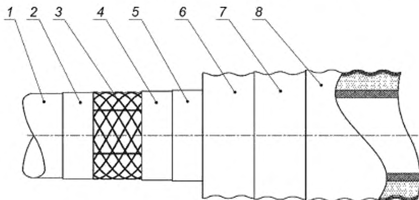
1 — внутренний слой; 2 — адгезионный слой; 3 — армирующий слой; 4 — наружный слой; 5 — барьерный слой (опционально); 6 — теплоизоляционный слой; 7 — барьерный слой (опционально); 8 — защитная оболочка
