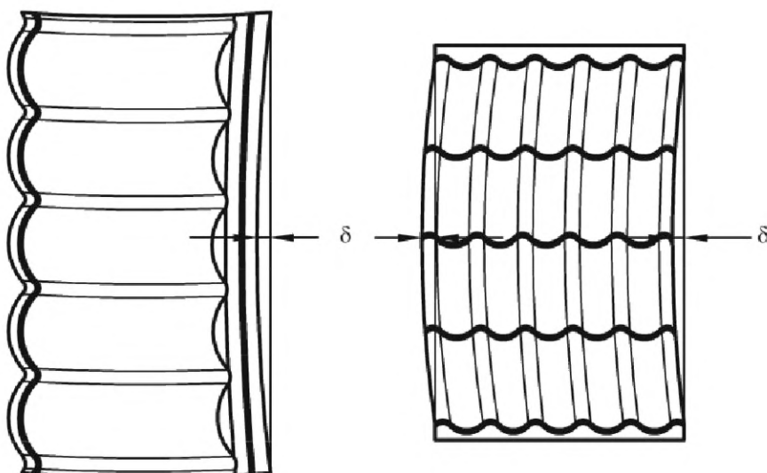
Рисунок 6 — Серповидность
