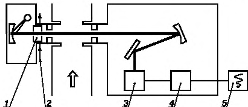
1 — хвост для калибровочных газовых смесей; 2 — впуск для калибровочных газовых смесей, 3 — приемник оптического излучения; 4 — блок электронной обработки данных; 5 — регистратор данных
