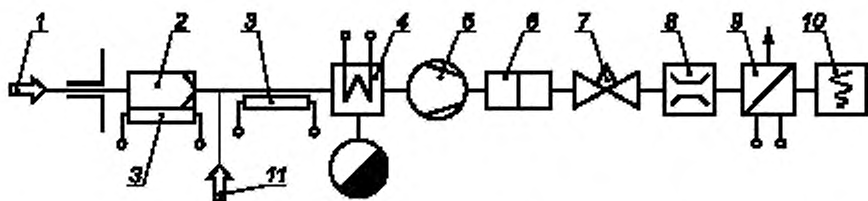
1 — зонд для отбора пробы; 2 — фильтр для удаления твердых частиц; 3 — нагревательная оболочка; 4 — охладитель пробы с сепаратором конденсата; 5 — насос для прокачивания пробы; 6 — фильтр; 7 — вентиль тонкой регулировки; 8 — расходомер; 9 — газоанализатор; 10 — регистратор данных; 11 — отверстие для ввода калибровочной газовой смеси, содержащей диоксид серы, и нулевого газа
