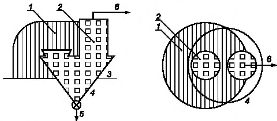
1 — зона класса 22, обычно радиусом в 1 м; 2 — зона класса 20; 3 — основание; 4 — загрузочная воронка для мешков, 5 — к электрооборудованию; 6 — в пылезащитную оболочку
