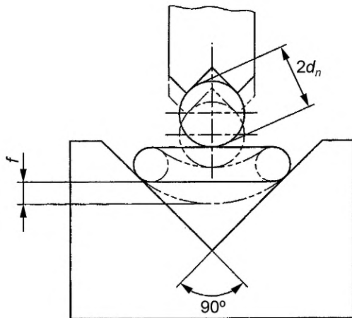
Рисунок 2 — Прогиб f
