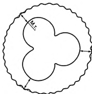
Рисунок 9 — Измерение толщины оболочки (наружная поверхность неправильной формы)
