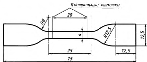
Рисунок 12 — Образец в виде двусторонней лопатки
