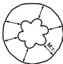
Рисунок 4 — Измерение толщины изоляции (многопроволочная жила)
