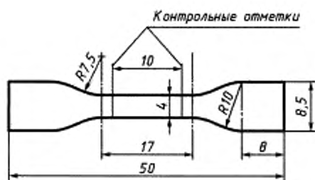
Рисунок 13 — Образец в виде двусторонней лопатки уменьшенного размера
