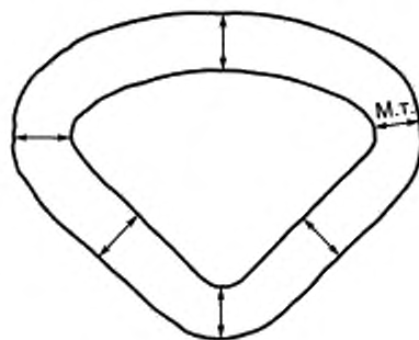
Рисунок 2 — Измерение толщины изоляции (секторная жила)
