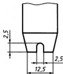
Рисунок 14 — Конеч вырубного ножа с выемкой
