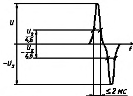
Рисунок 3 — Определение ширины импульса
