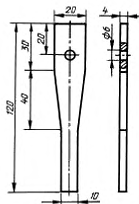
Рисунок 1.2 — Стальная пружина
