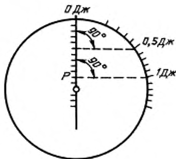
Рисунок 1.6 — Градуировка шкалы
