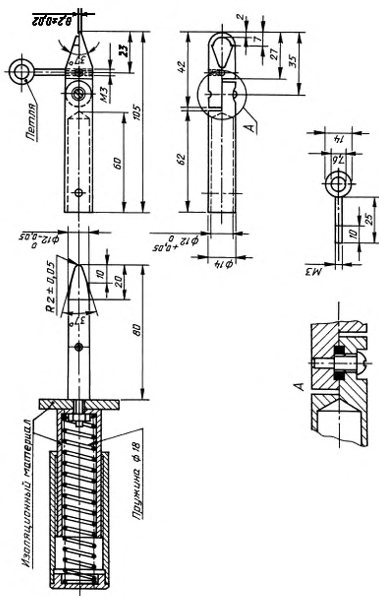
Рисунок 10 – Испытательный полураспределительный палец
