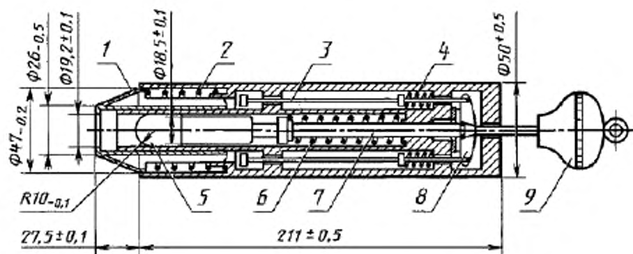
Устройство для испытания на удар
