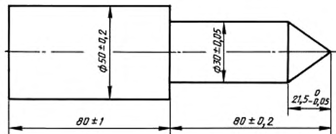
Рисунок 3 — Испытательный щуп
