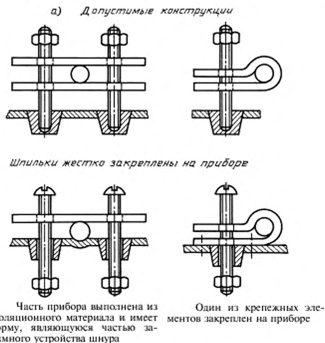
Рисунок 12 — Примеры выполнения крепления шнура. Лист 1
