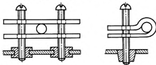
б) Недопустимые конструкции
