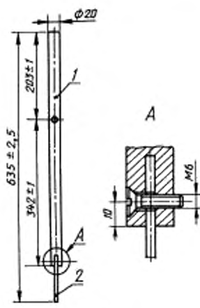
1 — сталь; 2 — пружина Рисунок 1.1 — Маятник
