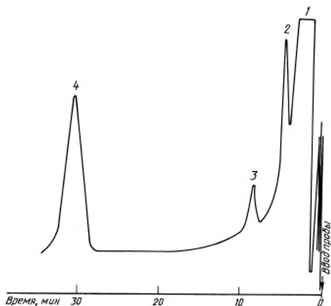
1 — 1,2-дихлорэтан; 2 — 1,1,2-трихлорэтан; 3 — додекан; 4 — 1,1,2,2-тетрахлорэтан
