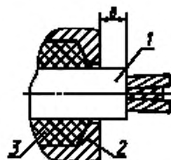
1 — оболочка кабеля; 2 — стенка вводного устройства; 3 — уплотнение
