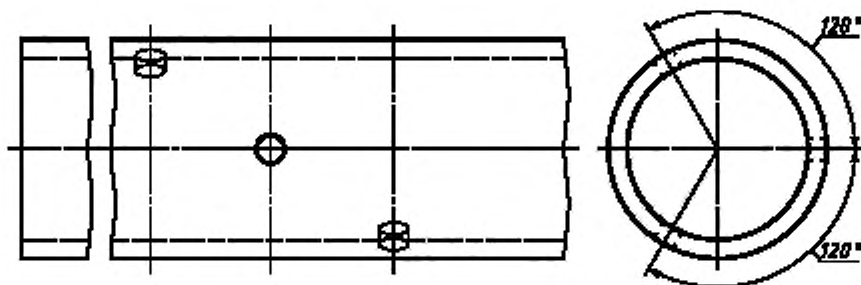
Рисунок В.1 — Эталонный образец с тремя отверстиями
