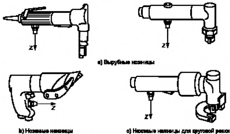
Рисунок 2 — Направления измерений и примеры размещения датчика вибрации
