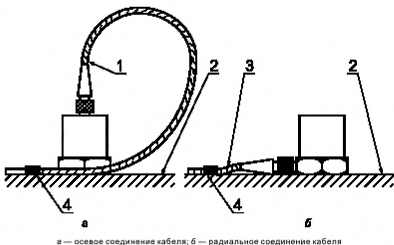
а — осевое соединение кабеля; б — радиальное соединение кабеля
