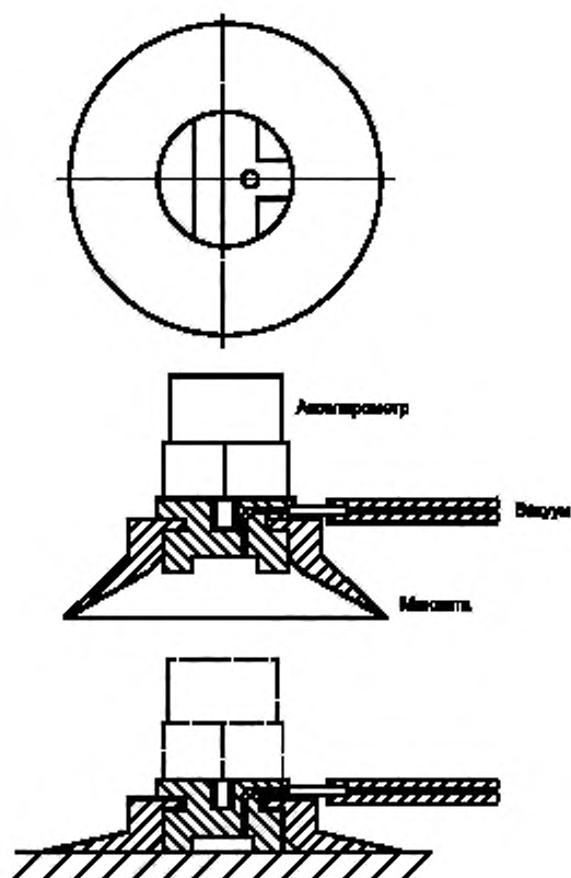
Рисунок 11— Вакуумное крепление
