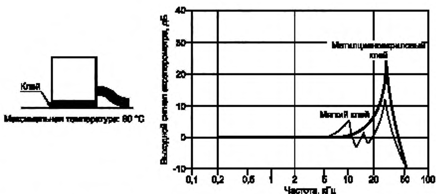
Рисунок 6 — Типичная частотная характеристика акселерометра при клеявом соединении
