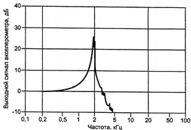
Рисунок 8 — Типичная частотная характеристика акселерометра с шупом
