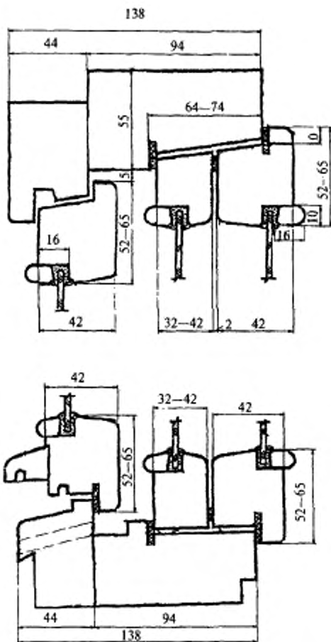
Рисунок 5 – Примеры конструктивных решений оконных блоков раздельно-спаренной конструкции
