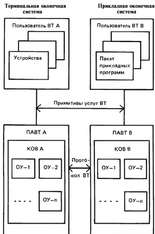
Рисунок 2 — Объекты управления в модели протокола ВТ
