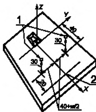
1 — микрофон; 2 — граница зоны измерений; w — ширина игрушки
