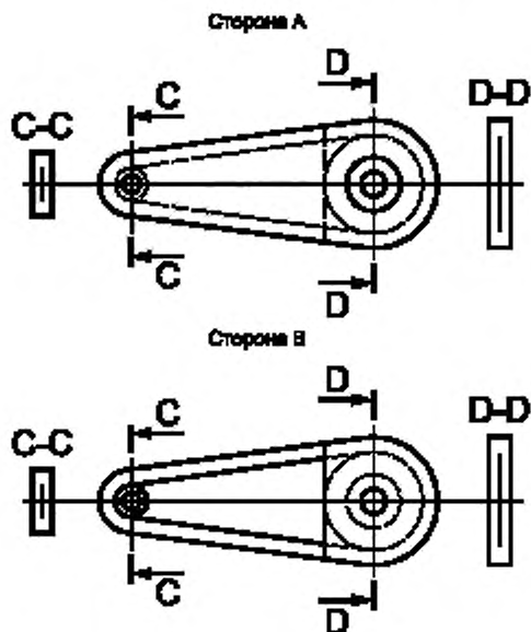
Рисунок 7 — Приводные цепи и защитные устройства цепи
