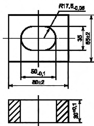
Рисунок 17 — Испытательный шаблон А
