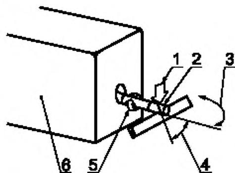
Рисунок 15 — Устройство для испытания кромок
