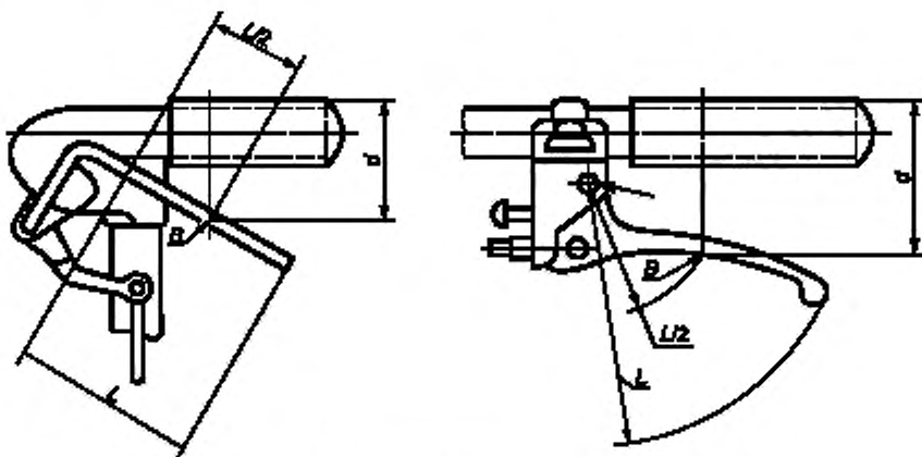
Рисунок 8 — Размеры рычага ручного тормоза
