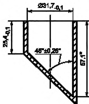
Рисунок 12 — Цилиндр для мелких деталей
