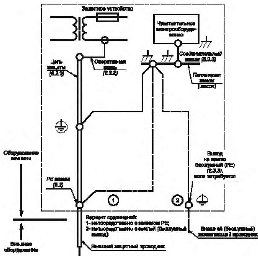
Рисунок 3 — Пример эквипотенциального соединения машины
