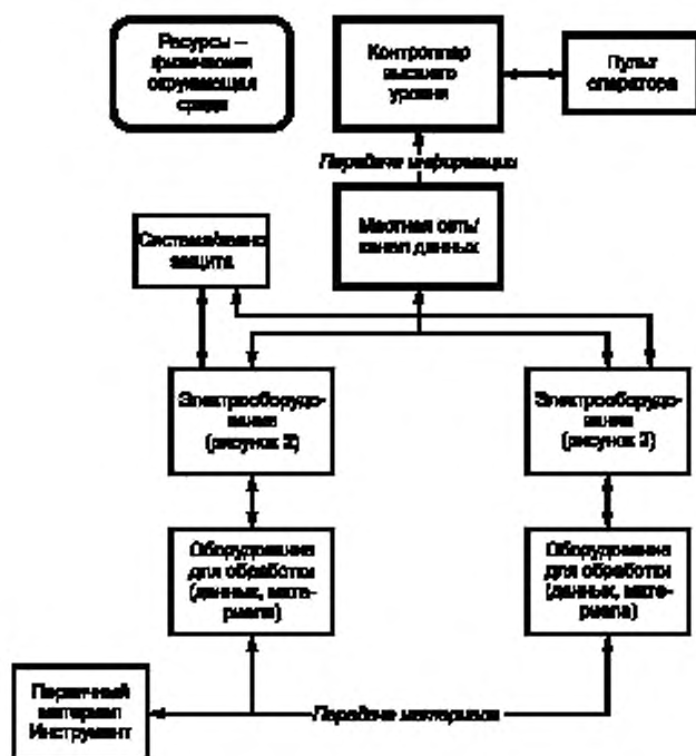
Рисунок 1 — Функциональная схема типовой производственной системы
