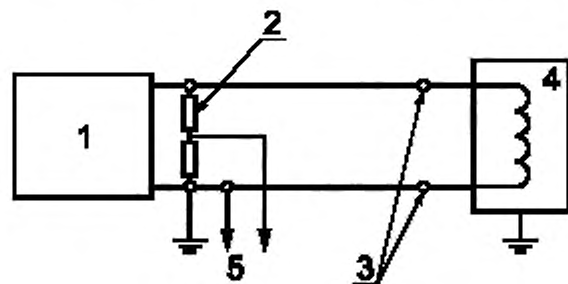
1 - генератор импульсов; 2 - делитель напряжения; 3 - соединительные контактные зажимы; 4 - испытываемое балластное устройство; 5 - контактные зажимы для присоединения электронного осциллографа
