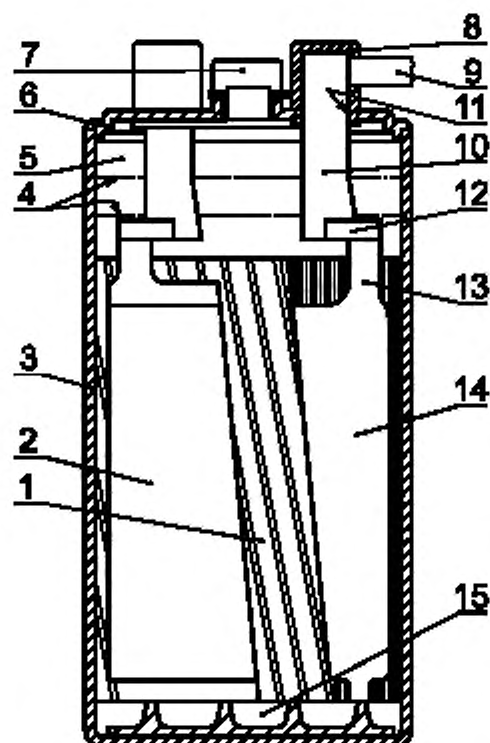
1 – сепаратор; 2 – положительная пластина; 3 – корпус; 4 – уровень электролита (макс./мин.); 5 – свободное пространство; 6 – уплотнение крышки, непроницаемое для электролита; 7 – заглушка в отверстии для заливки; 8 – уплотнение полюсного штыря; 9 – перемычка; 10 – полюсный штырь; 11 – уплотнение полюсного штыря; 12 – гребенка; 13 – выступ аккумуляторной пластины; 14 – отрицательная пластина; 15 – Пространство для отложения шлама
