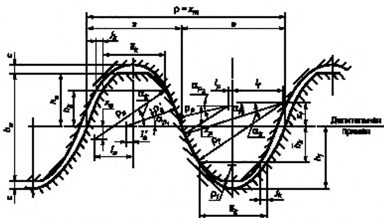
Рисунок 1 — Исходный контур
