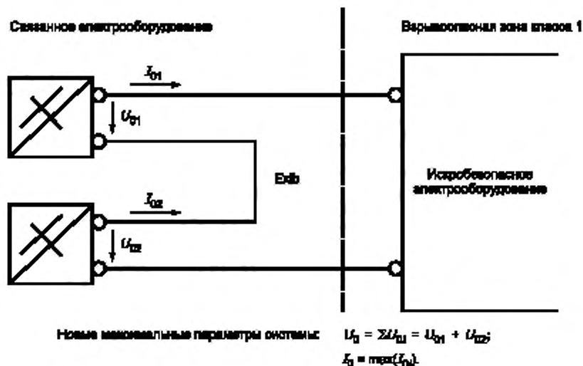
Рисунок В.1 — Последовательное соединение. Суммирование напряжений
