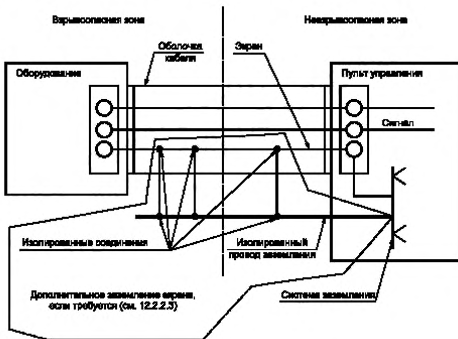
Рисунок 2 — Заземление проводящих экранов
