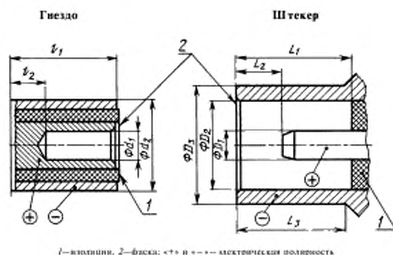
Рисунок 1—Гнездо и штекер теплельного соединителя
