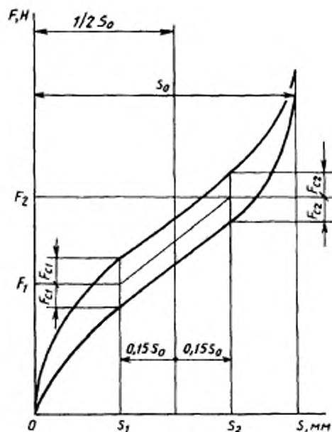
Рисунок 2 — Упругая характеристика сиденья
