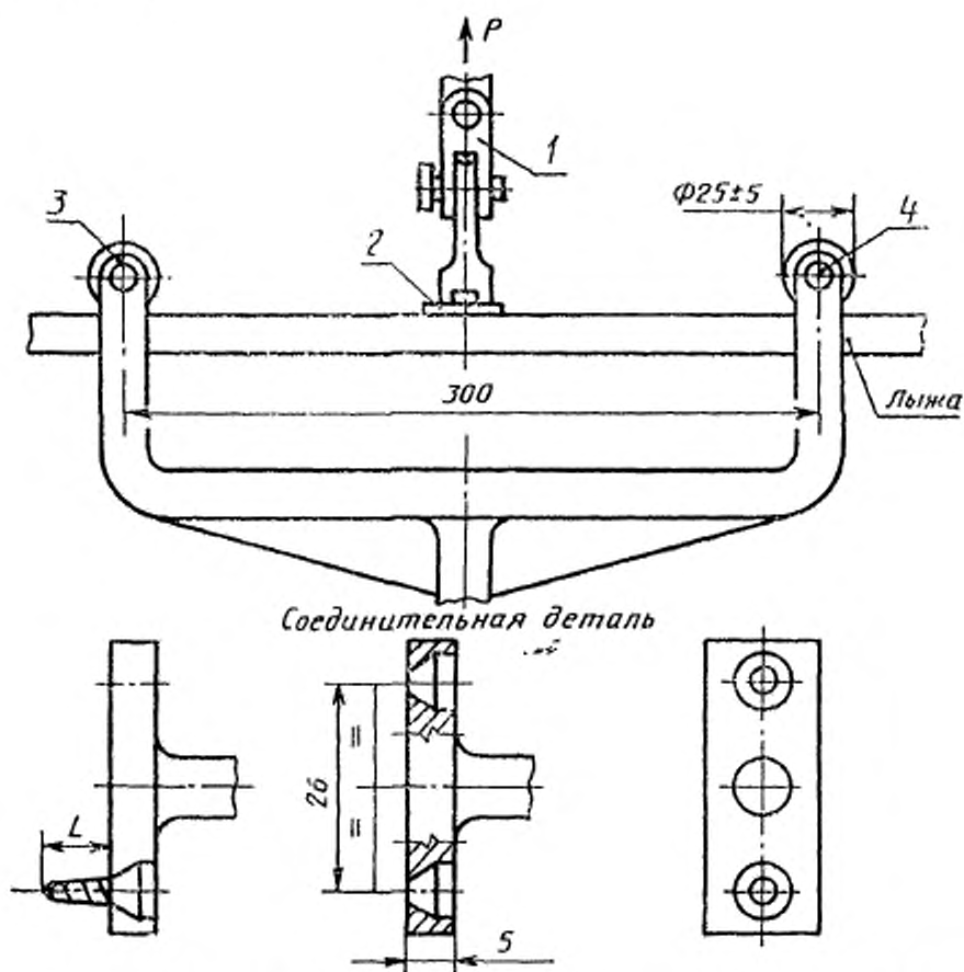
1 — зажимное приспособление испытательной машины; 2 — соединительная деталь; 3 — опора; 4 — свободновращающаяся точка опоры (валок); L — глубина проникания шурупа
