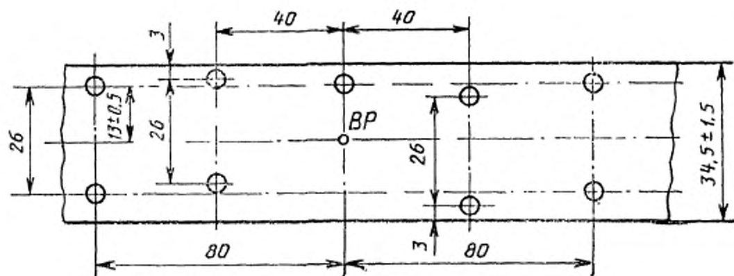
Рисунок 7 — Соединительная деталь
