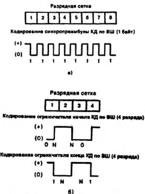
Рисунок 8 — Кодирование синхропреамбулы и ограничителей начала и конца КД
