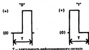
Рисунок 2 — Представление информации в НШ при использовании ВОСРП
