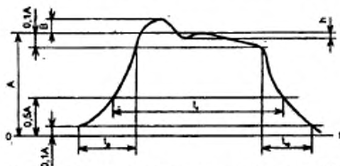
Рисунок 12 — Форма сигнала оптического излучения в ВОСРП
