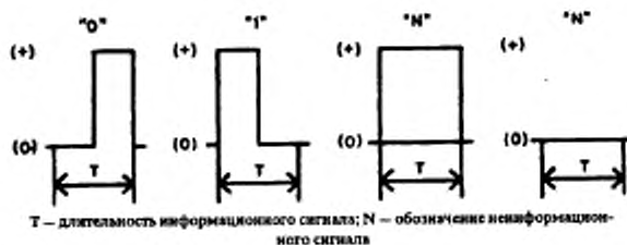
Рисунок 3 — Представление информации в ВШ
