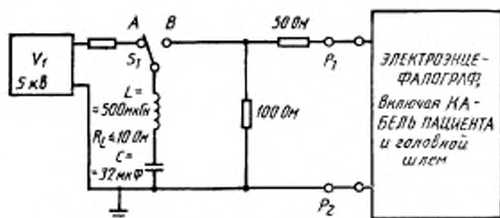
Рисунок 102 — Испытание защиты от воздействия разряда кардиодефибриллятора (см. 51.101 настоящего стандарта)
