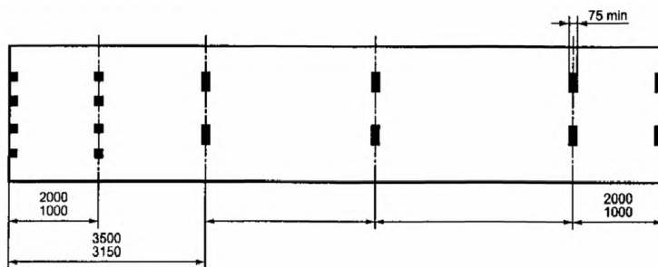
Рисунок Б.4 – Минимальное количество пар опорных (контактных) площадок контейнеров типов 1AAA, 1AA, 1A и 1AX с тоннелем для захвата типа «шея гуся»
