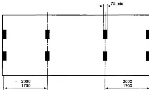
Рисунок Б.2 – Минимальное количество пар опорных (контактных) площадок контейнеров типов 1ССС, 1С и 1СХ (при наличии) и контейнеров типов 1ВВВ, 1ВВ, 1В и 1 ВХ
