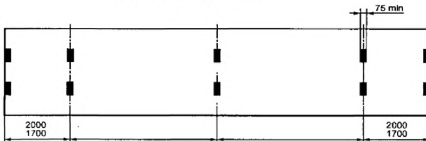
Рисунок Б.3 – Минимальное количество пар опорных (контактных) площадок контейнеров типов 1ААА, 1АА, 1А и 1АХ без тоннеля для захвата типа «шея гуся»
