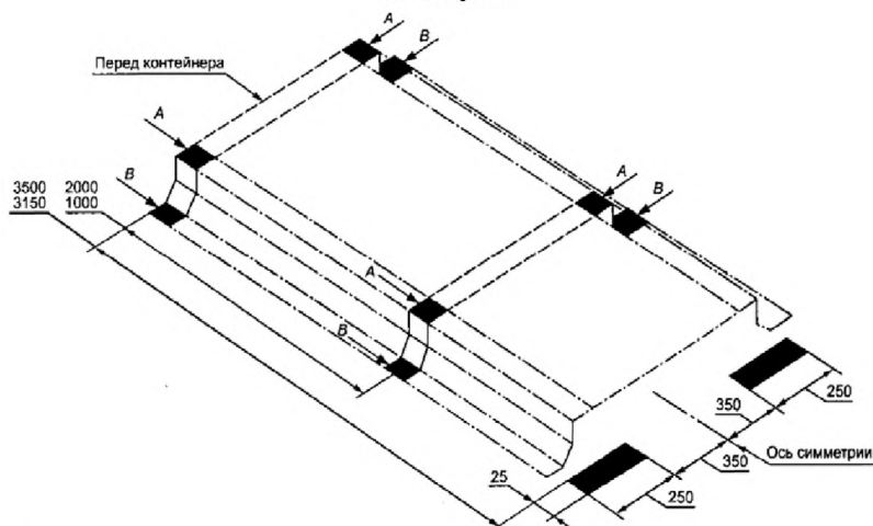
Рисунок Б.4 – Минимальное количество пар опорных (контактных) площадок контейнеров типов 1AAA, 1AA, 1A и 1AX с тоннелем для захвата типа «шея гуся»
