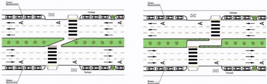
Рисунок 4.8. Варианты велосипедного перехода в одном уровне со смещением
