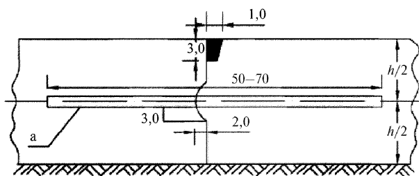
а – стержень-анкер
