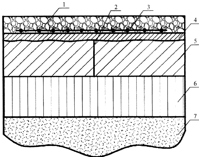
1 – слой усиления из асфальтобетона; 2 – деформационный шов; 3 – геосетка; 4 – выравнивающий слой; 5 – старое цементобетонное покрытие; 6 –основание; 7 – грунт земляного полотна Рисунок 9 – Усиление цементобетонного покрытия асфальтобетоном с использованием геосетки с устройством выравнивающего слоя
