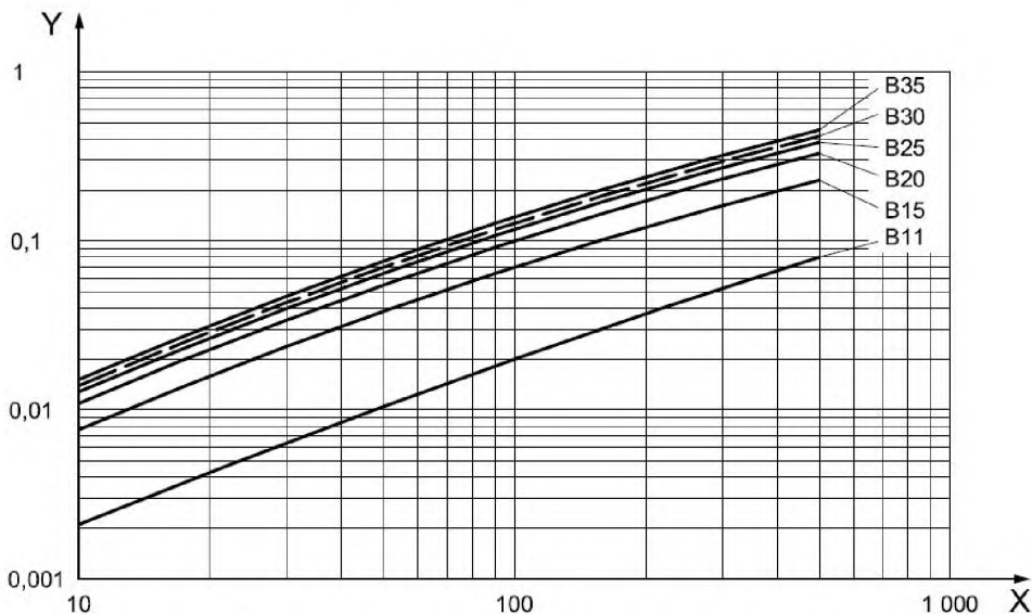
Рисунок С.1 – Зависимость между коэффициентом индуктивной связи k , длиной цепи связи и диаметром жгута проводов в случае испытательных импульсов, имитирующих медленные переходные процессы
