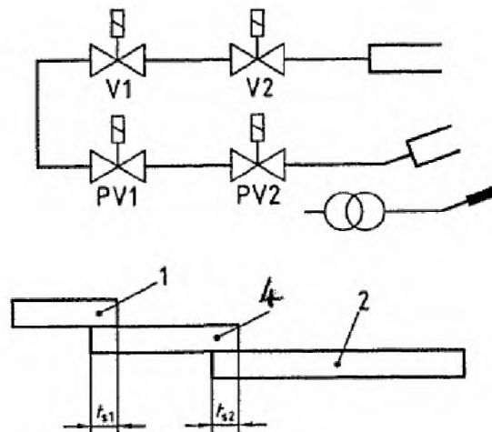
Рисунок 10 – Прямой розжиг основной горелки при пониженной нагрузке с независимой подачей газа при розжиге
