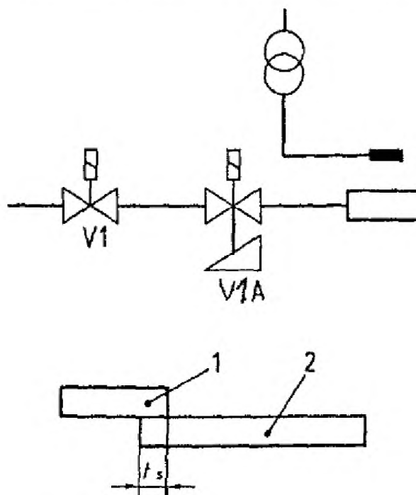
Рисунок 8 – Прямой розжиг основной горелки при максимальной мощности
