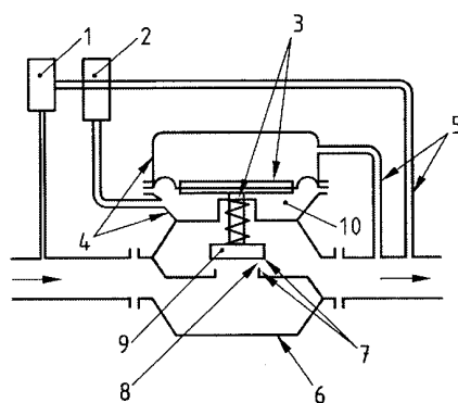
Рисунок А.1 – Пример регулятора прямого действия
