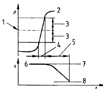
Рисунок С.6 – Измерение времени срабатывания
