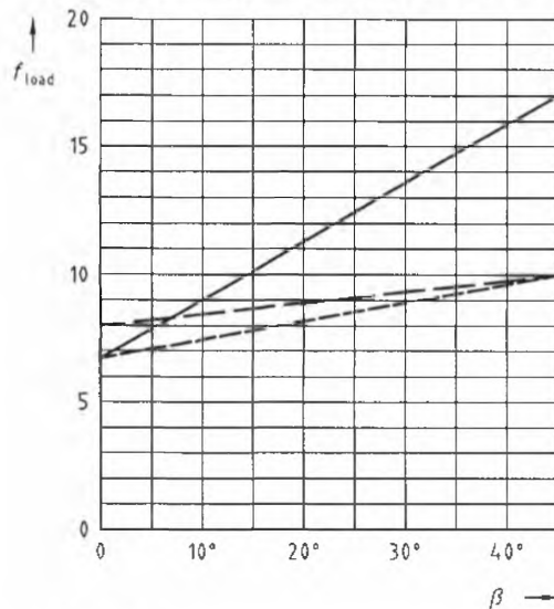
Рисунок 9 – Винтовое анкерное крепление
