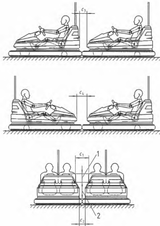
Рисунок 32а – Атракционный электромобиль
