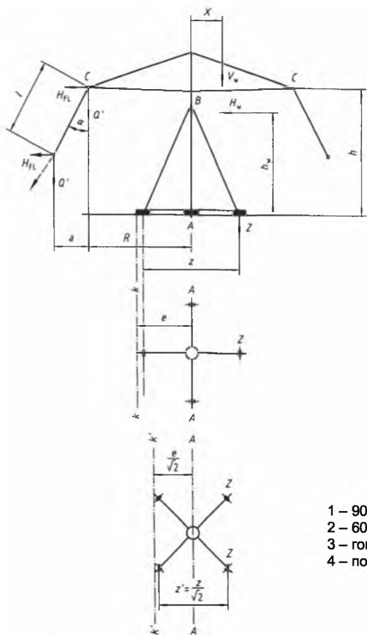
Рисунок В.5а – Маховик карусели (вид сбоку)
