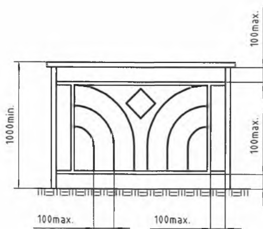
Рисунок 16 – Ограждения с декоративными встроенными элементами
