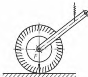
Рисунок 34 – Усилие контакта между поверхностью пола и щеткой
