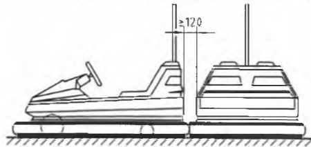
Рисунок 19 – Безопасное расстояние для свободно движущихся транспортных средств
