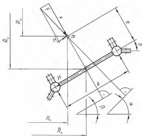
Рисунок 7 – Поперечное сечение рельсов с опорными и направляющими колесами
