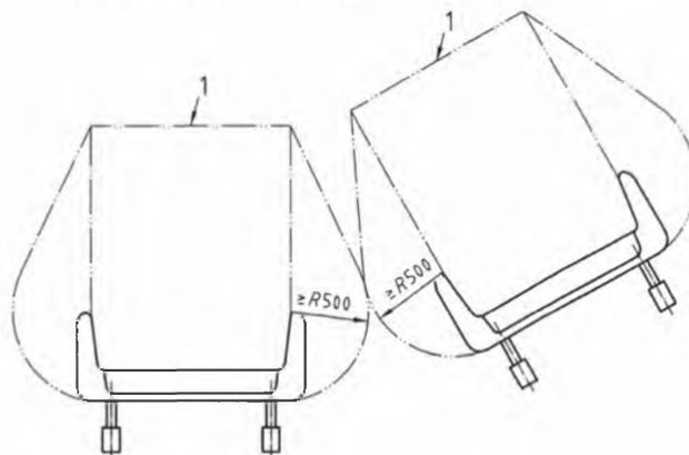
Рисунок 20 – Ограничение расположения контуров свободного пространства
