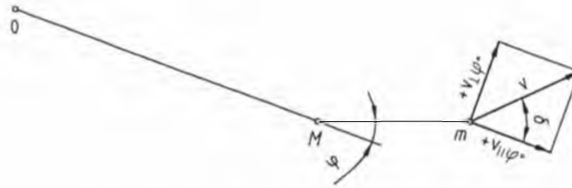
Рисунок 4 – Составляющие скорости v
