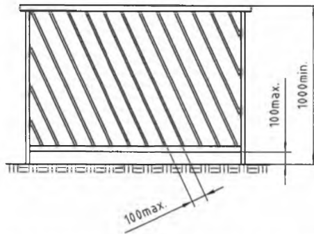
Рисунок 14 – Ограждение со преимущественно вертикальными встроенными элементами
