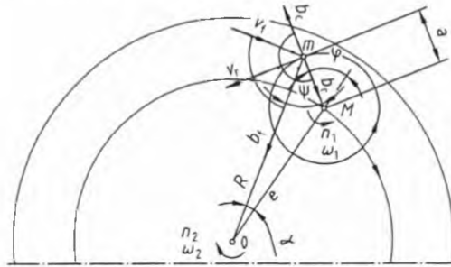
Рисунок 3 – Скорость и ускорение центра материальной точки m
