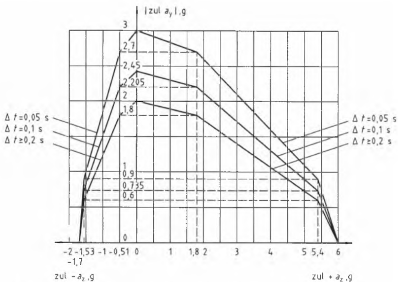
Рисунок G.5 – Допустимые ускорения a_y и a_z при совместном воздействии
