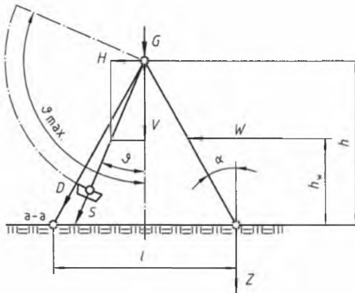
Рисунок В.1 – Качели «Лодка»
