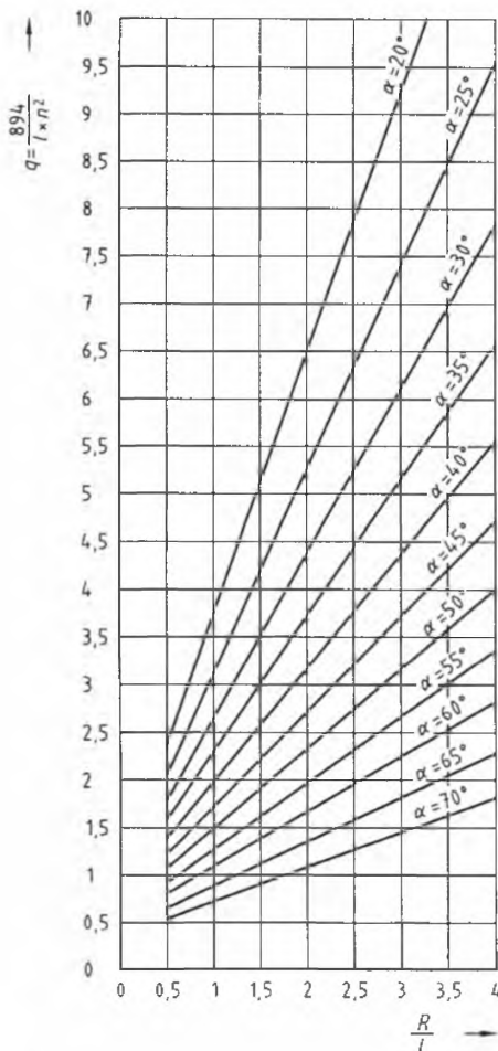
Рисунок В.4 – Номограмма для определения угла отклонения \alpha
