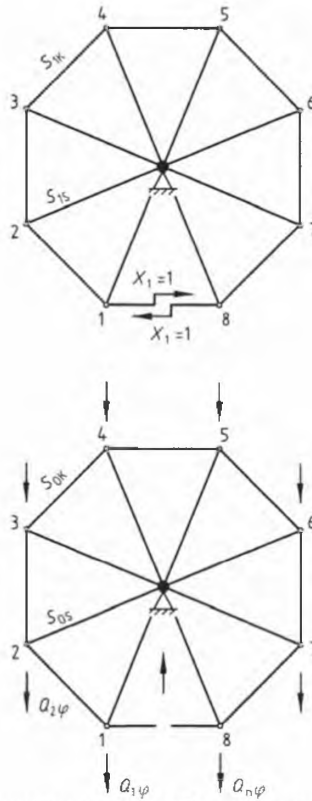
Рисунок В.3 – Статически неопределенная базовая система колеса обозрения с n = 8 секторами (многоугольная компоновка)
