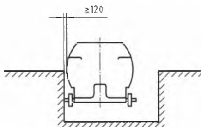
Рисунок 35 – Минимальное расстояние до стены канала
