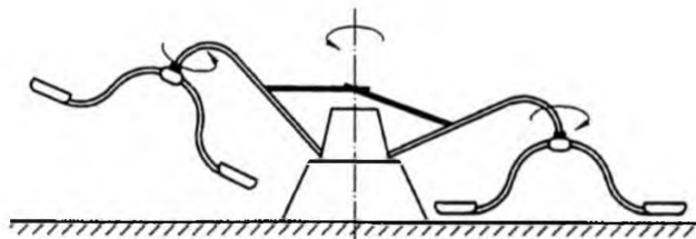
Рисунок 26 – Оси, изменяющие наклон
