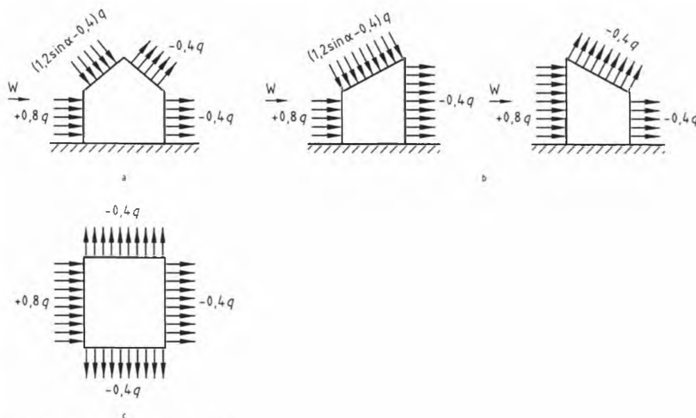
Рисунок 1 – Аэродинамические коэффициенты для конструкций обычной формы
