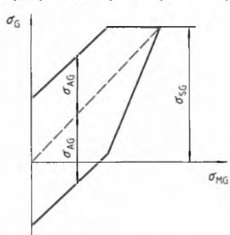
Рисунок 12 – Диаграмма предела усталости согласно теории Смита в зависимости от формы
