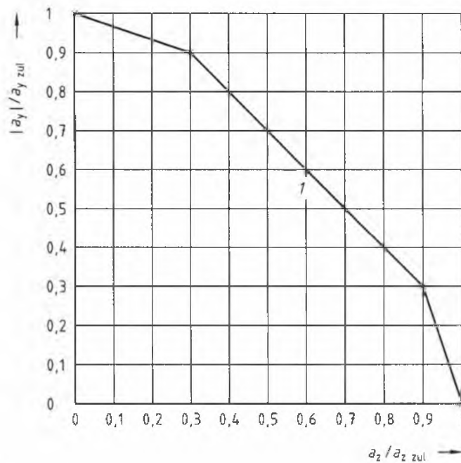
Рисунок G.4 – Совместное воздействие ускорений |a_y| и |a_z|
