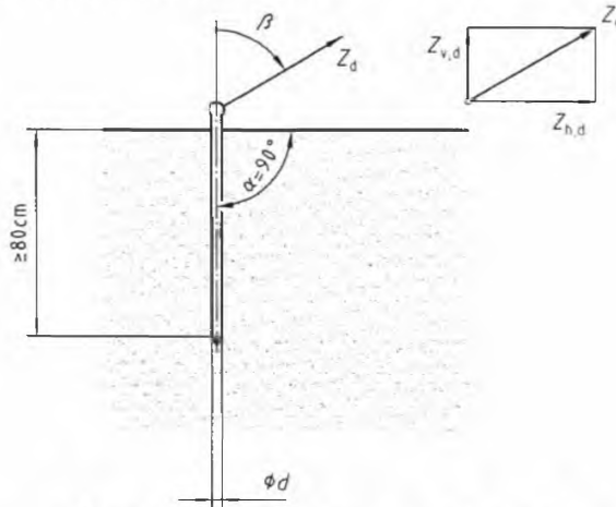
Рисунок 9 – Винтовое анкерное крепление
