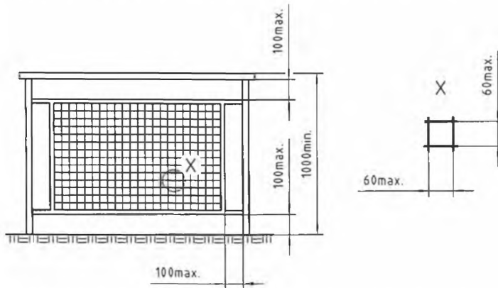
Рисунок 15 – Ограждения со встроенной сеткой или панелями
