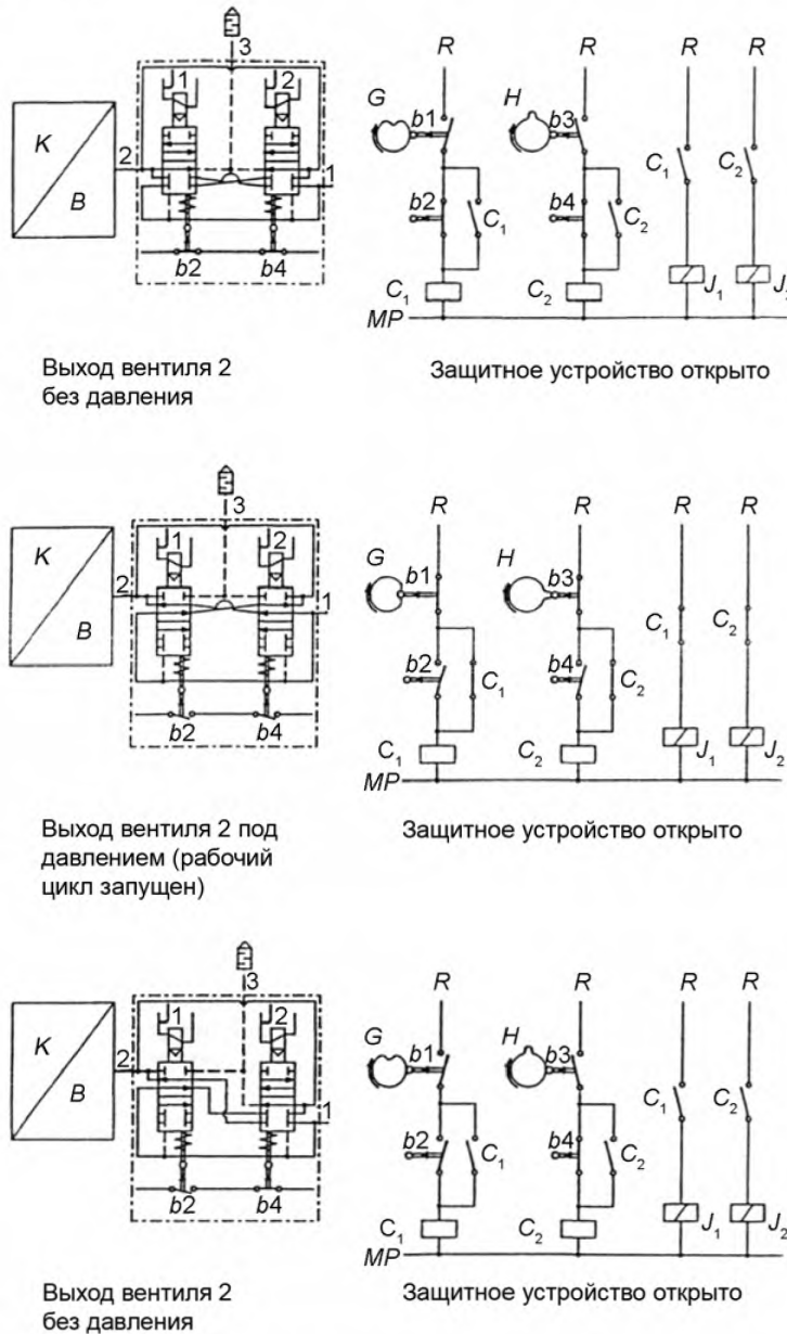
Рисунок В.2 – Образец схемы переключения к рисунку В.1
