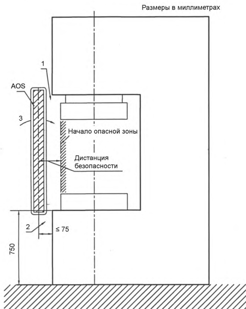
Рисунок. Е.1 – Пример типичного применения используемого для запуска цикла AOS на прессе для грузочных работ (боковые разделительные защитные устройства на этом рисунке не представлены)
