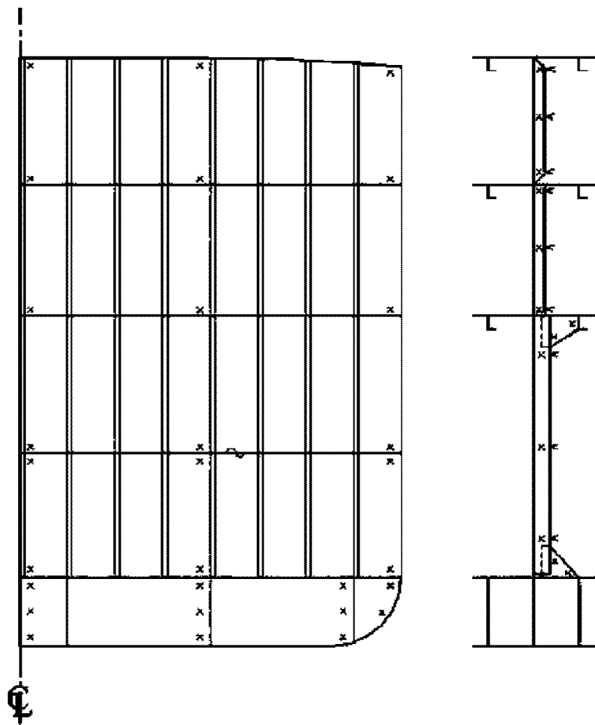
Рис. 5.3.1-2 Схема замеров толщин обшивки плоских поперечных переборок с вертикальными р.ж.
