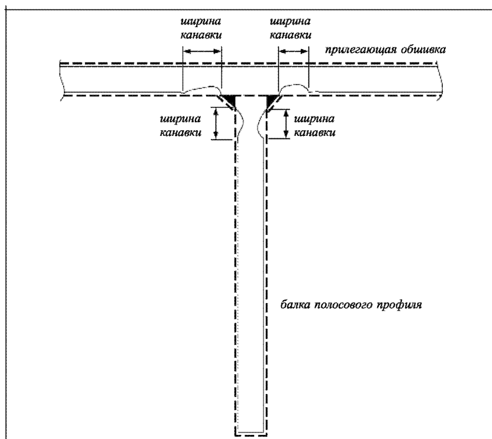
Рис. 1.2.1-4 Канавочный износ
