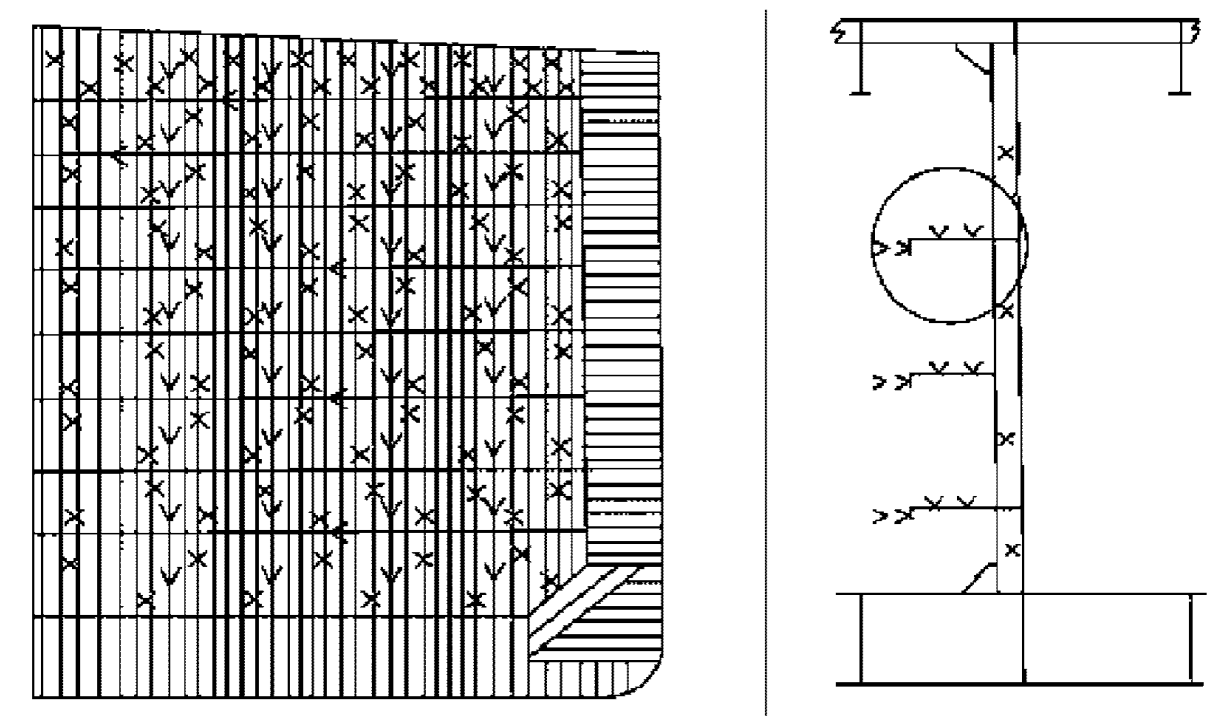
Рис. 5.3.1-3 Схема замеров поперечных переборок грузовых танков нефтеналивного судна с двойными бортами и двойным дном
