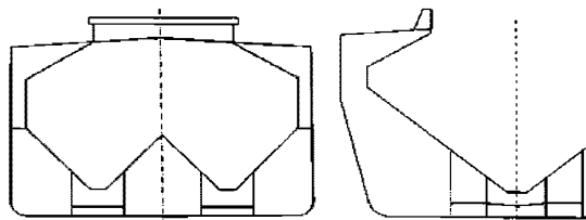
Рис. 2.2.9 Типовые сечения мидель-шпангоута саморазгружающегося навалочного судна
