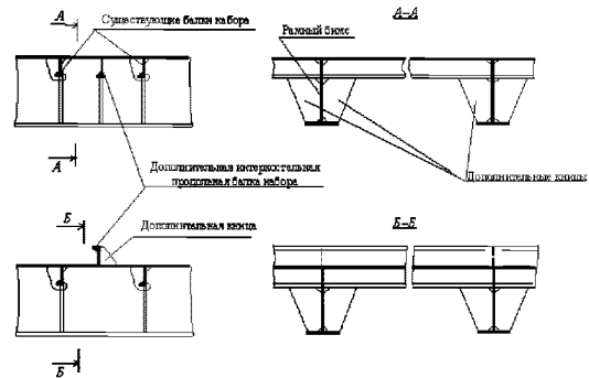
Рис. 5.2.2.5-2 Установка дополнительных балок набора
