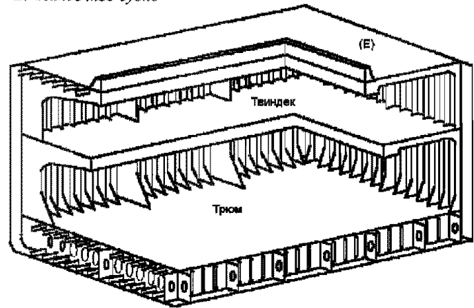
Рис. 7.2.3.2-1 Районы А, В и Е детального освидетельствования судов, предназначенных для перевозки сухих генеральных грузов
