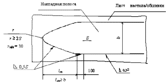
Рис. 5.2.1.3-2 Оформление окончаний накладных полос
