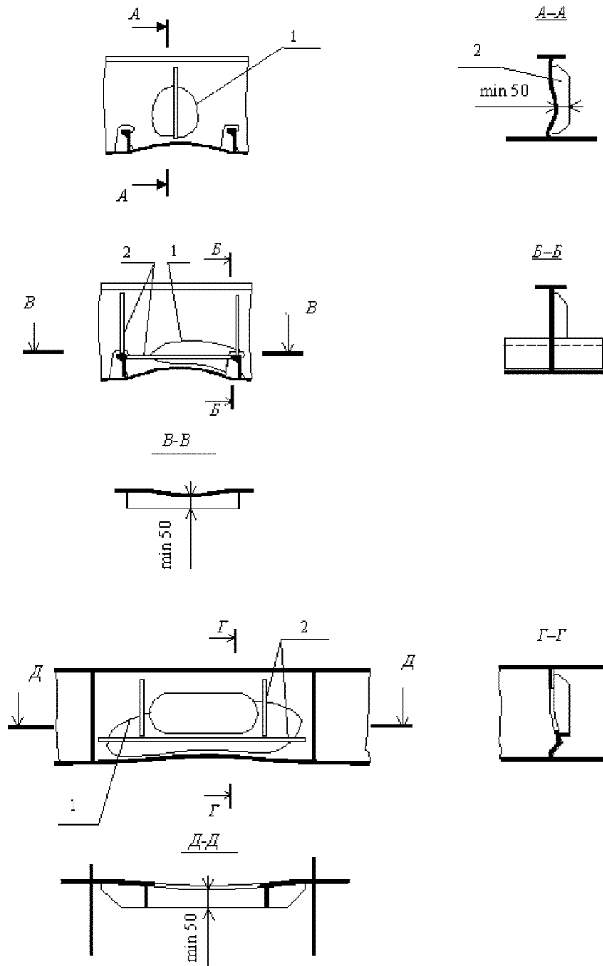
Рис. 5.3.4.2-2 Подкрепления выпучин: 1 — контур выпучины; 2 — ребро жесткости
