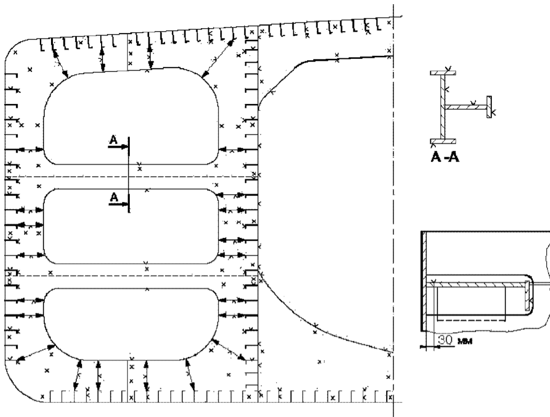
Рис. 5.3.1-12 Схема замеров поперечных рам однокорпусных нефтеналивных судов
