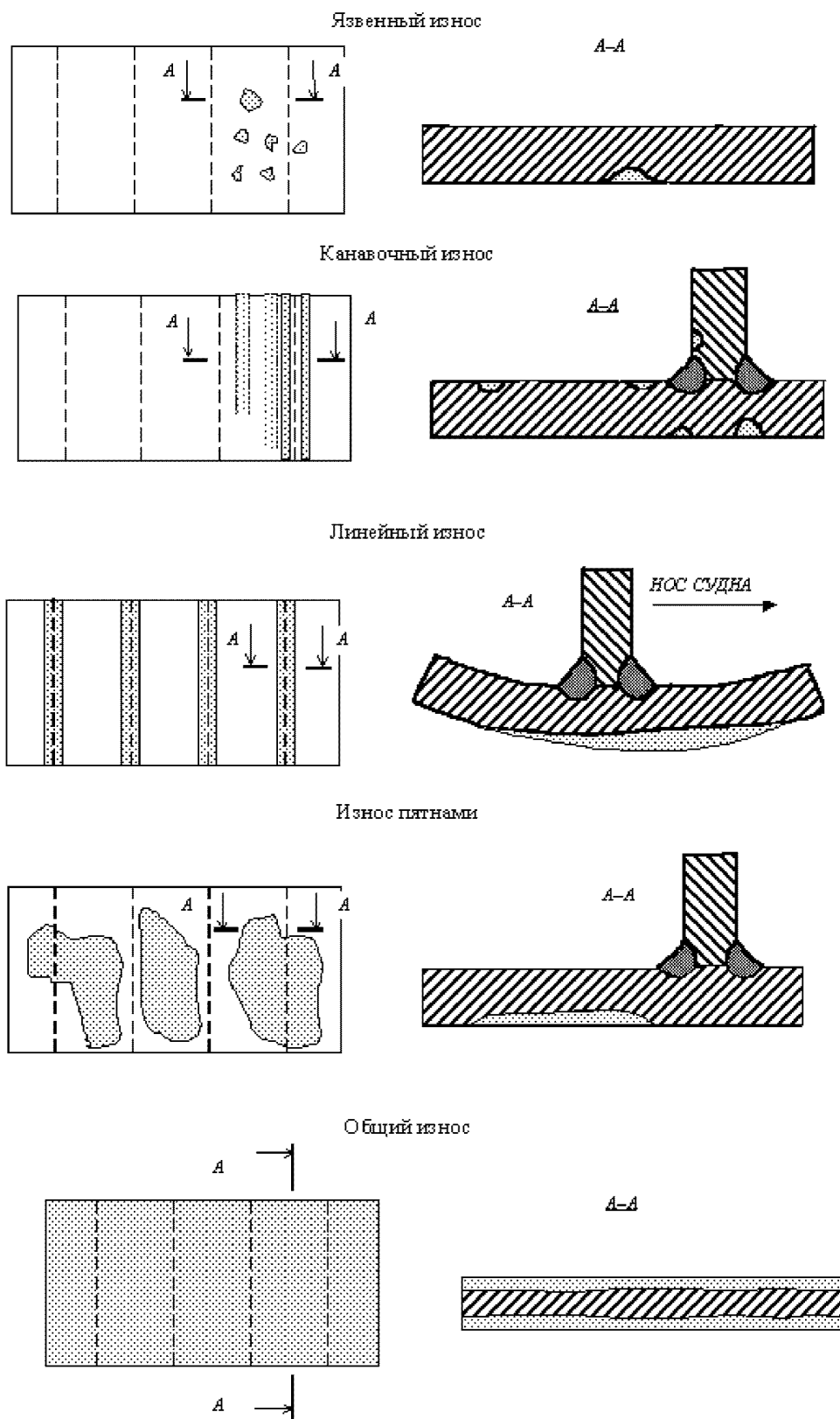
Рис. 1.2.1-2 Виды износов
