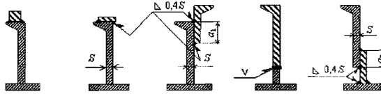
Рис. 5.2.4.1-1 Подкрепления балок набора:
