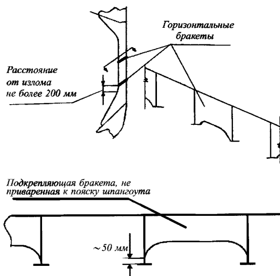
Рис. 5.12.3.3.1 Подкрепляющие бракеты
