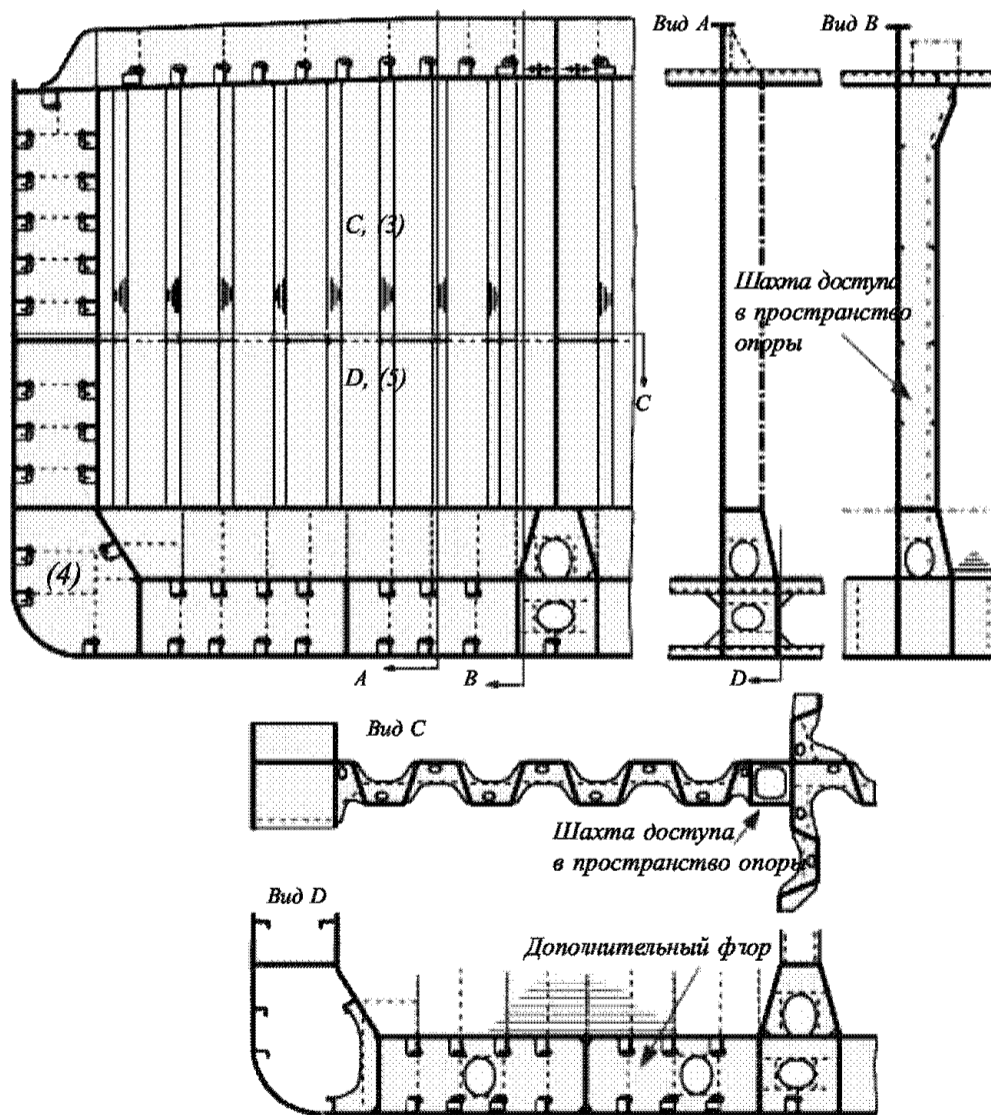
Рис. 4.2.3.2-1 Районы А и В, 1 и 2 деталей освидетельствований химовозов
