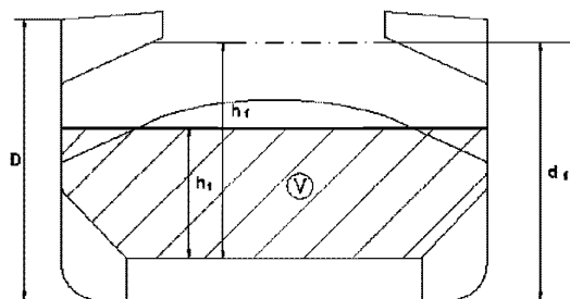
Рис. 5.10.2.2 Схема загруженного трюма ( V — объем груза, \text{м}^3 )
