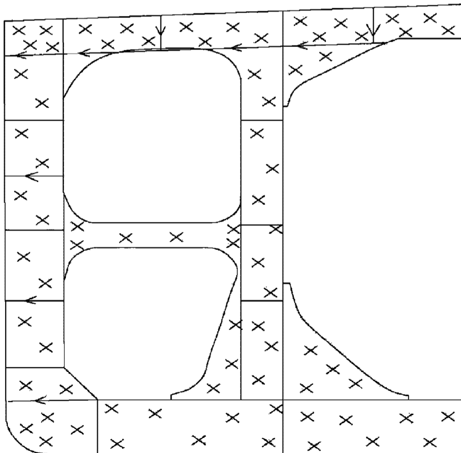
Рис. 5.3.1-13 Схема замеров поперечных рам нефтеналивных судов с двойными бортами и двойным дном
