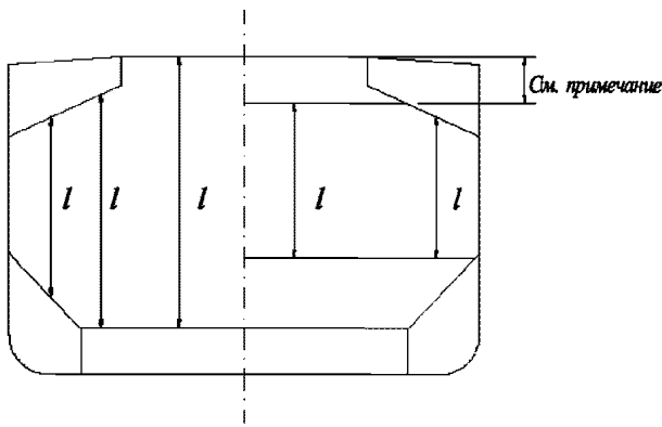
Рис. 5.9.3.1 Схема для определения пролета гофров поперечной переборки
