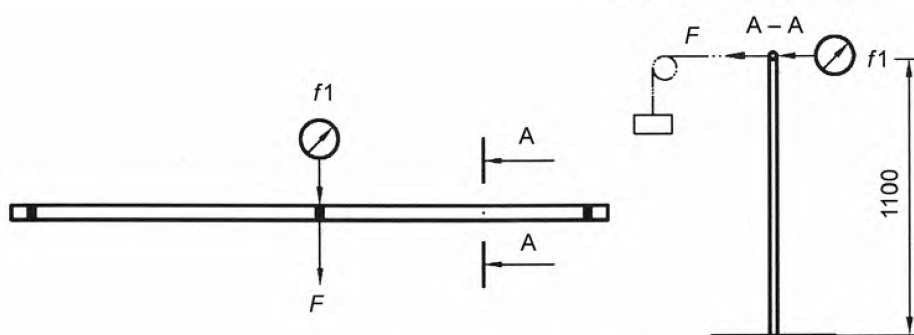
Рисунок 10 – Измерение стойки
