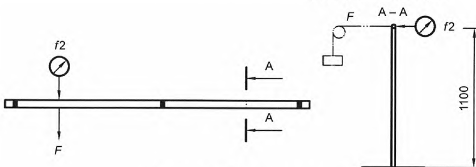
Рисунок 11 – Измерение поручня
