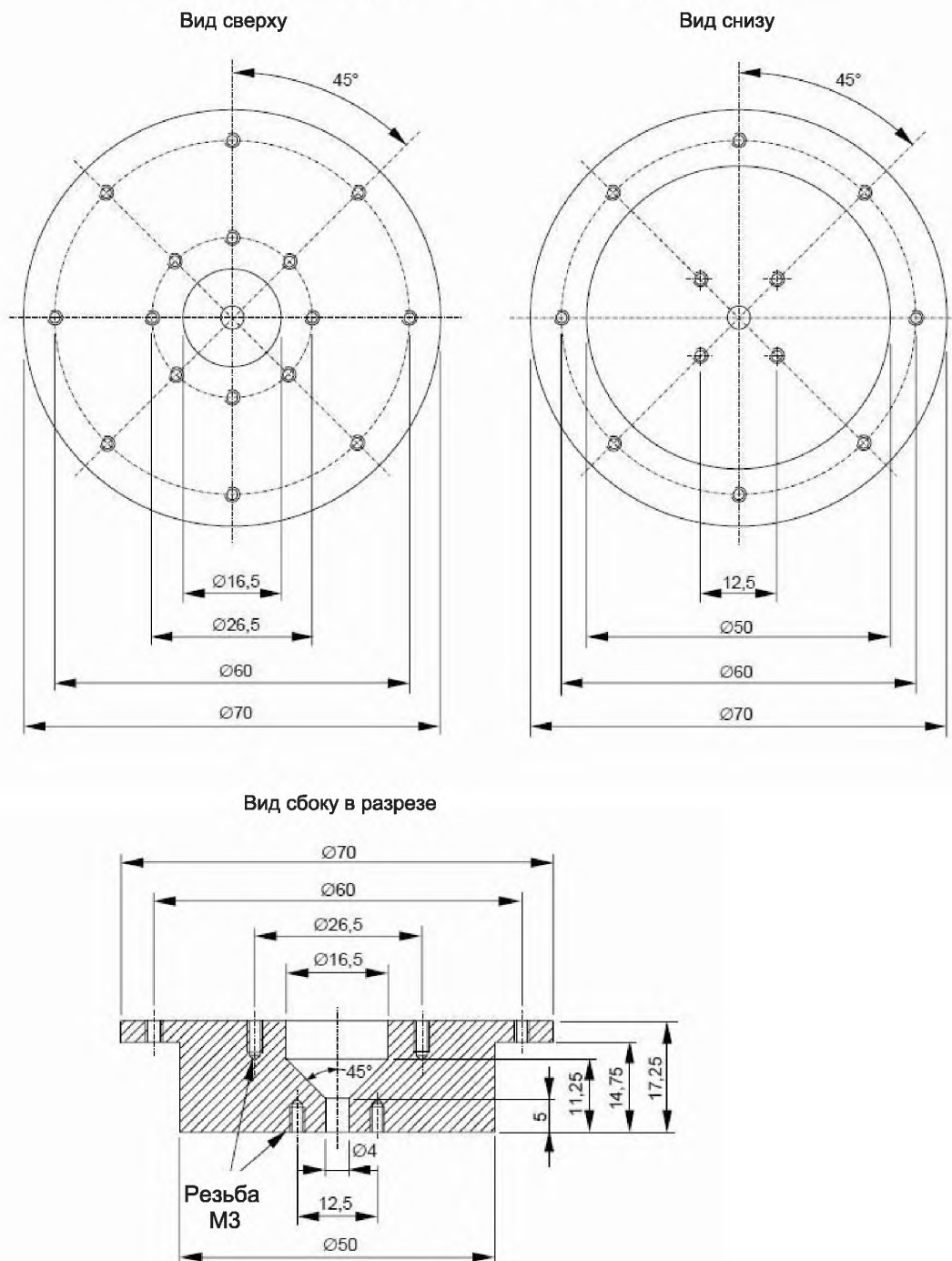
Рисунок С.1 – Сборочный чертеж коаксиального датчика (рисунок 1 из 5)
