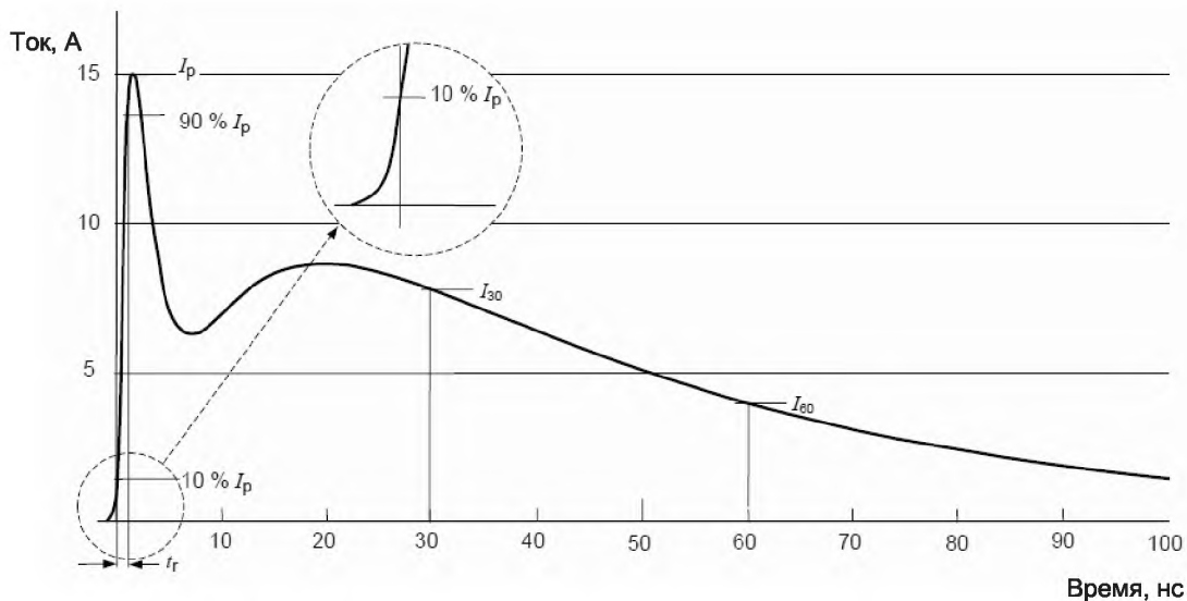
Рисунок 2 – Идеальная форма импульса разрядного тока при контактном разряде 4 кВ
