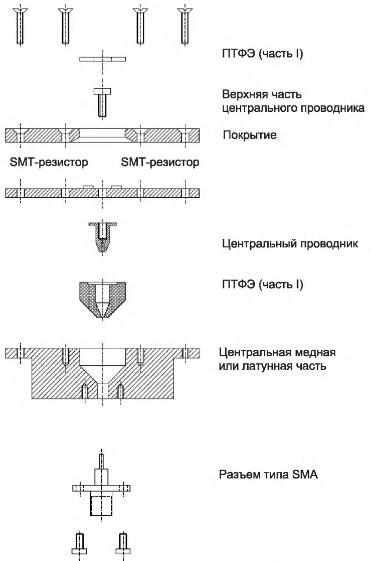
Рисунок С.5 – Сборочный чертеж коаксиального датчика (рисунок 5 из 5)
