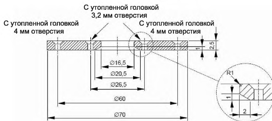
Рисунок С.4 – Сборочный чертеж коаксиального датчика (рисунок 4 из 5)
