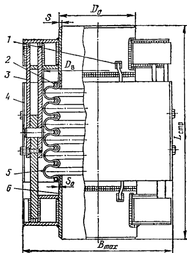
Рис. 3. Компенсатор односекционный волнистый осевой типа КВО на P_y=25 и 64 \text{ кгс/см}^2 ;
