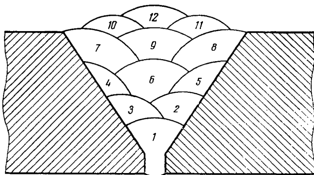
Рис. 12. Порядок заварки швов труб из сталей типа 15X5М аустенитными электродами.
