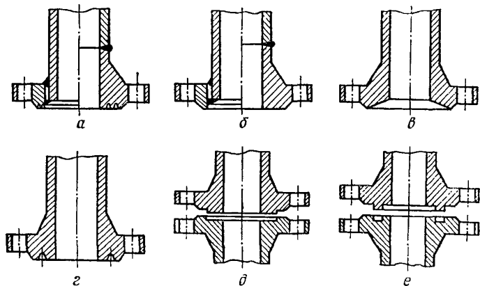
Рис. 1. Уплотнительные поверхности фланцев арматуры и соединительных частей трубопроводов:
