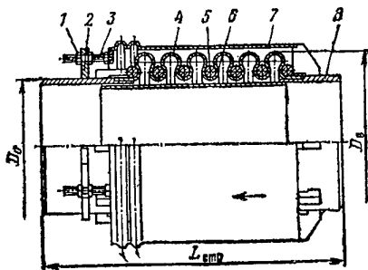
Рис. 3. Компенсатор односекционный волнистый осевой типа КВО на P_y=25 и 64 \text{ кгс/см}^2 ;
