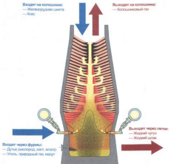
Рисунок 2.25 — Принципиальная технологическая схема работы доменной печи [52]
