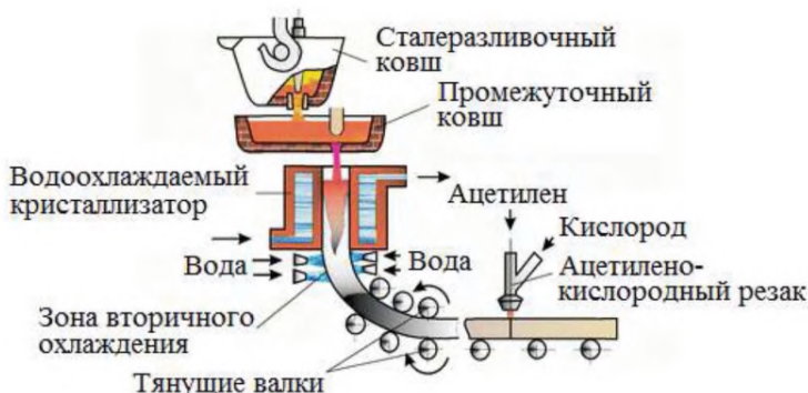
Рисунок 2.42 — Устройство МНЛЗ криволинейного типа
