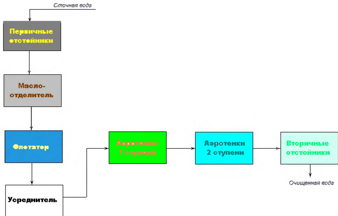
Рисунок 2.24 — Схема биохимической очистки сточных вод
