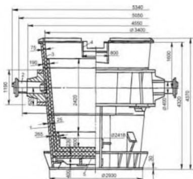
Рисунок 2.70 — Ковш сварной футерованный разливочный емкостью 20 м 3
