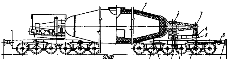
Рисунок 2.34 — Чугуновозный ковш миксерного типа
