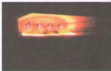
Рис. 6.1. Работа горелок ГНП.Р-250-31 горна агломашины
