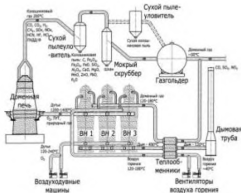
Рисунок 5.3 — Технологическая схема утилизации тепла дымовых газов
