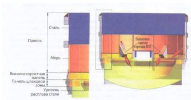
Рисунок 7.20 — Принципиальная конструкция электродуговой печи ULTIMATE
