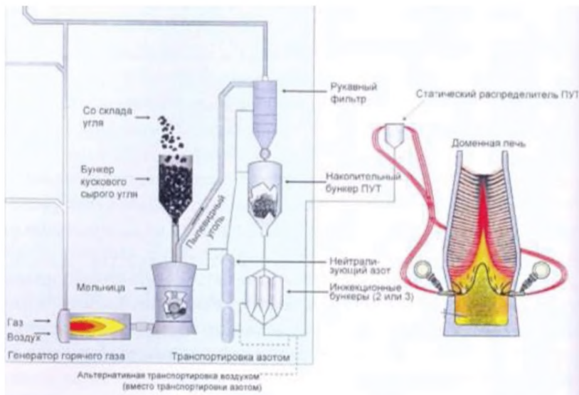
Рисунок 5.2 — Принципиальная схема установки подготовки и подасы ПУТ
