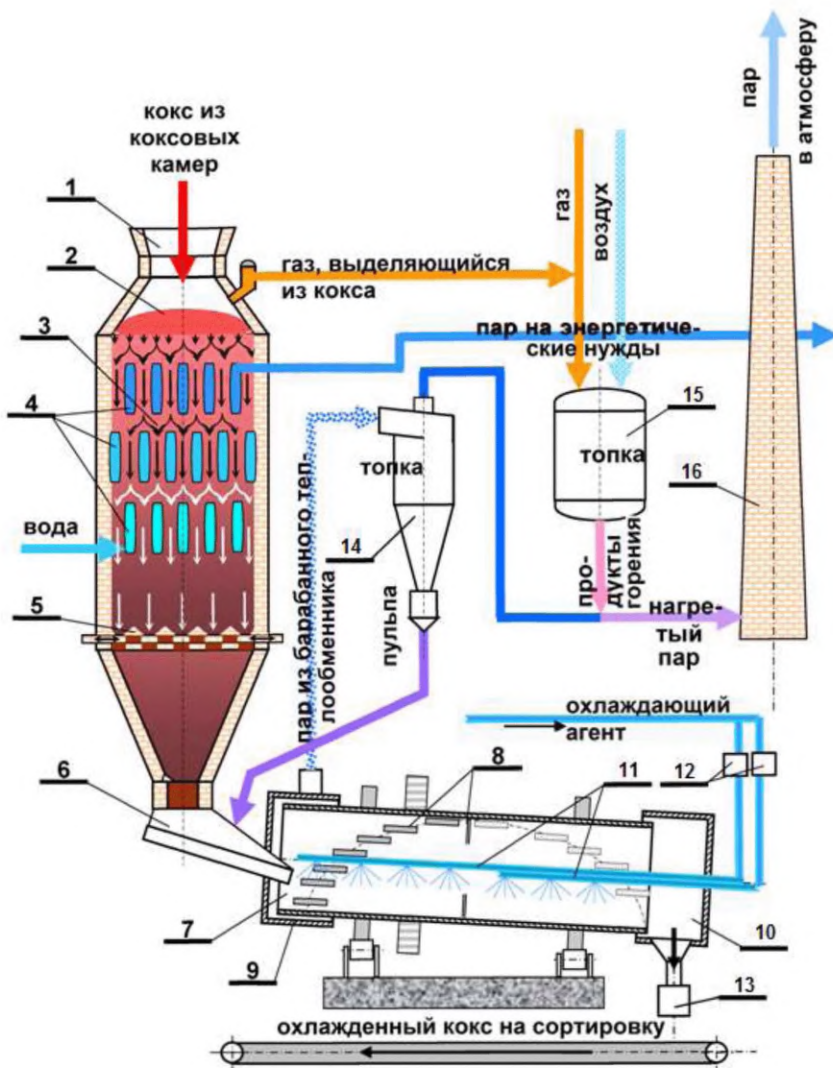
Рисунок 7.10 — Схема технологии ступенчатого охлаждения кокса
