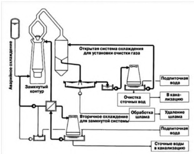
Рисунок 3.11 — Обратная схема водоснабжения доменного цеха [113]
