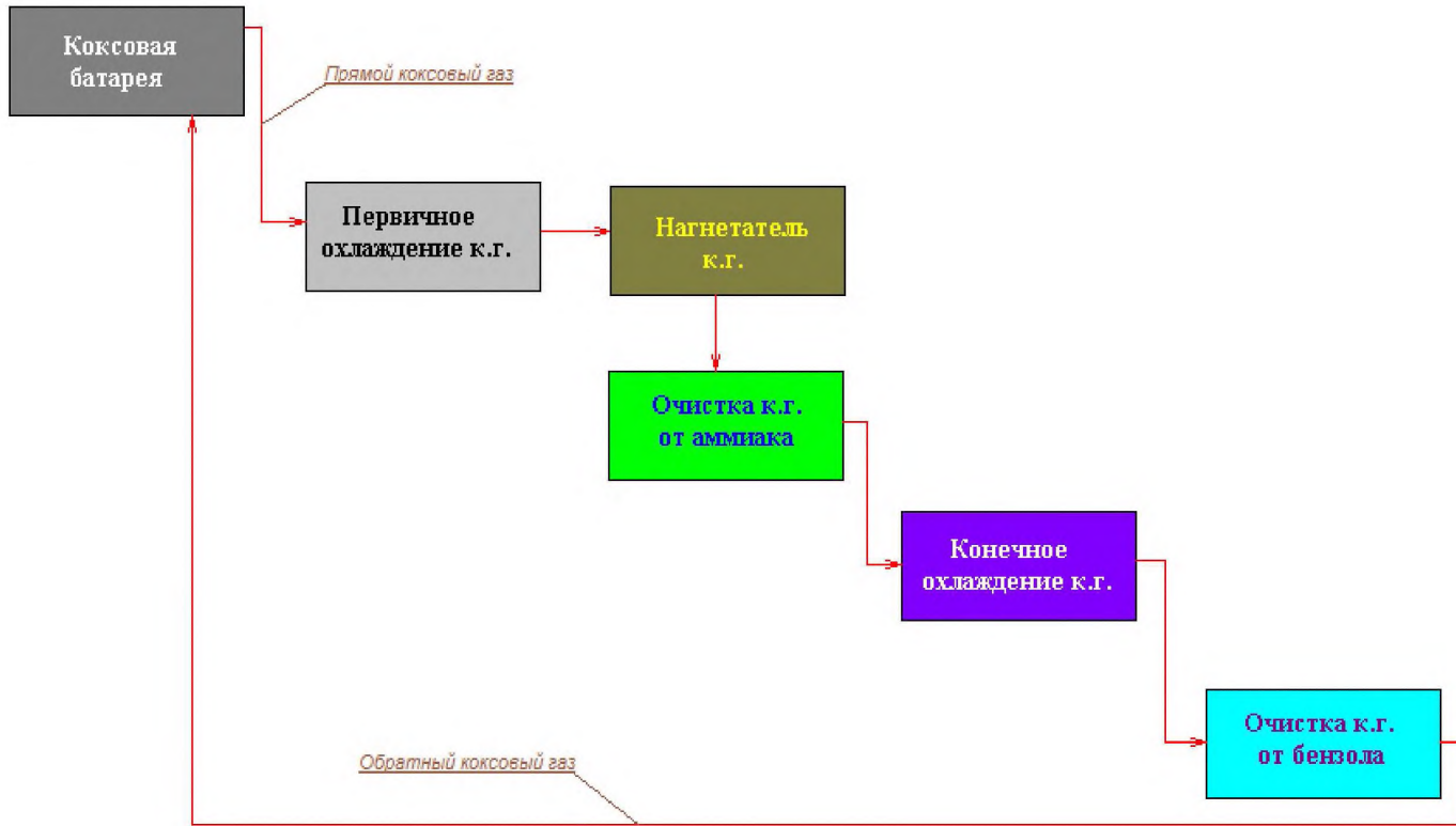
Рисунок 2.23 — Технологическая схема отделения конденсации цеха улавливания (пример)
