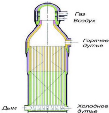
Рисунок 2.33 — Воздухонагреватель конструкции Я. П. Калугина
