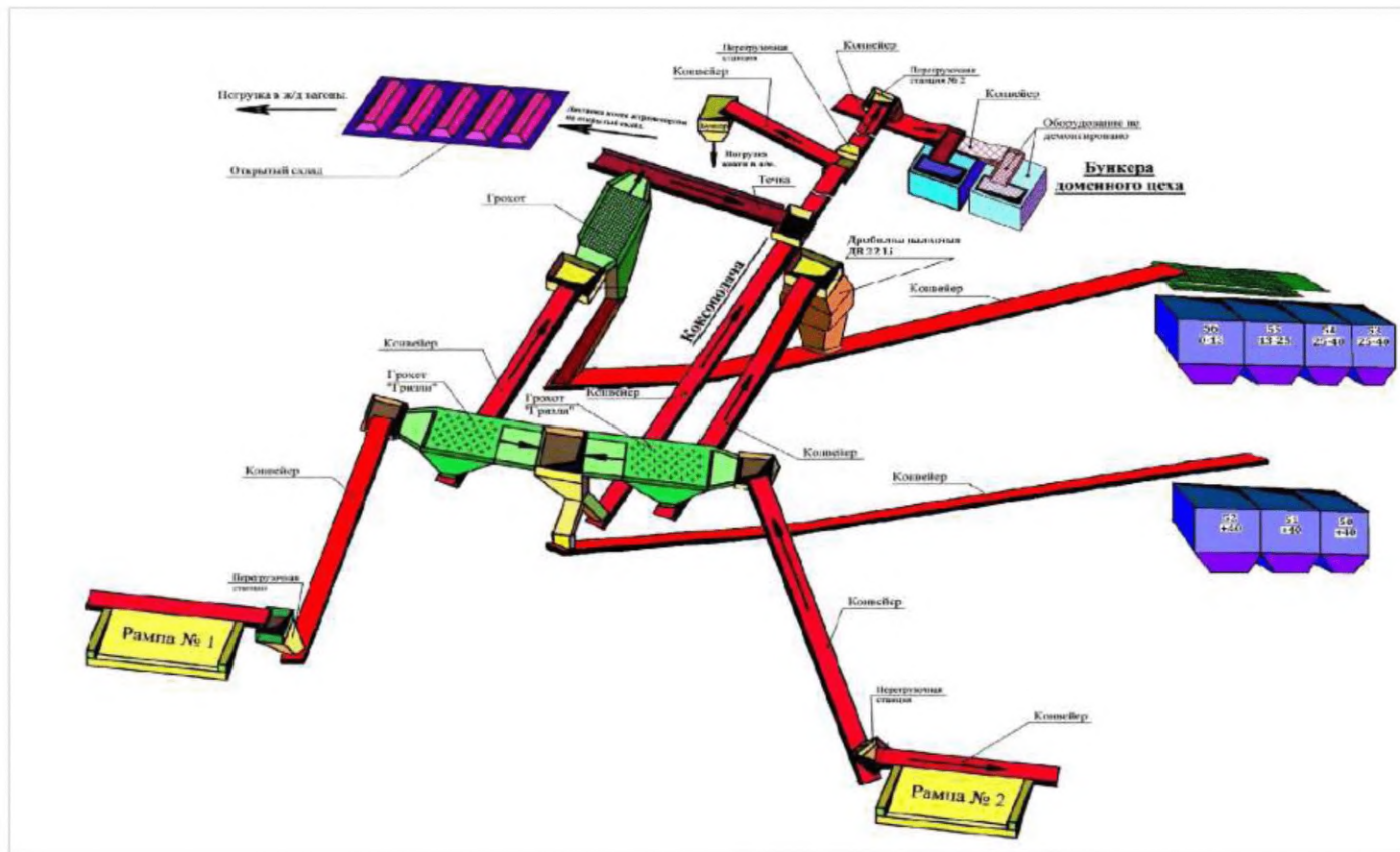
Рисунок 2.21 — Технологическая схема коксортировки (пример)
