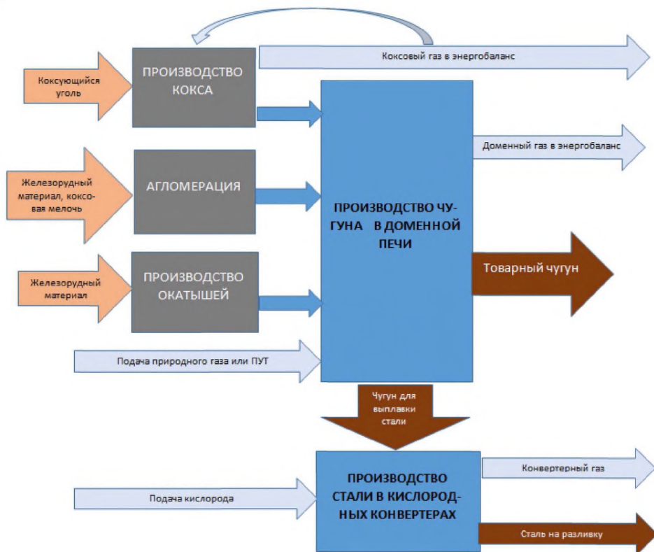
Рисунок 3.1 — Основные технологические процессы при производстве чугуна и стали [112]
