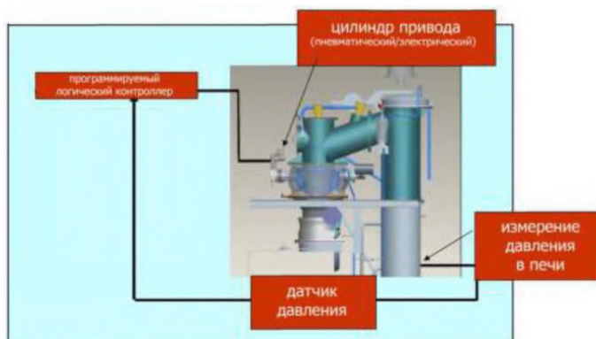
Рисунок 7.9 — Клапан SOPREKO
