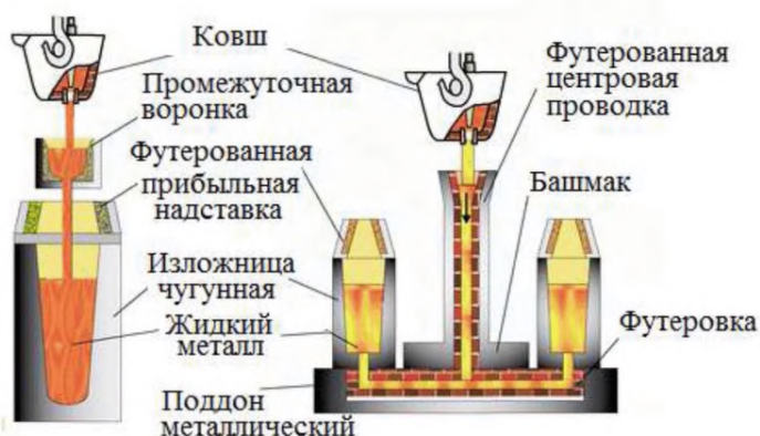
Рисунок 2.43 — Разливка стали в изложницы (слитки)
