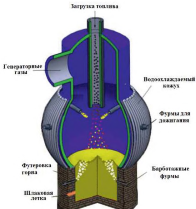
Рисунок 7.15 — Политопливный газогенератор конструкции НИТУ «МИСиС» [174]
