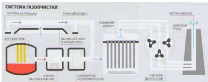
Рисунок 2.58 — Принципиальная схема пылегазоочистки с рукавным фильтром
