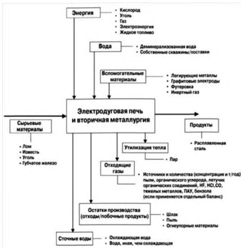
Рисунок 3.16 — Блок-схема материальных потоков в электродуговых печах [113]
