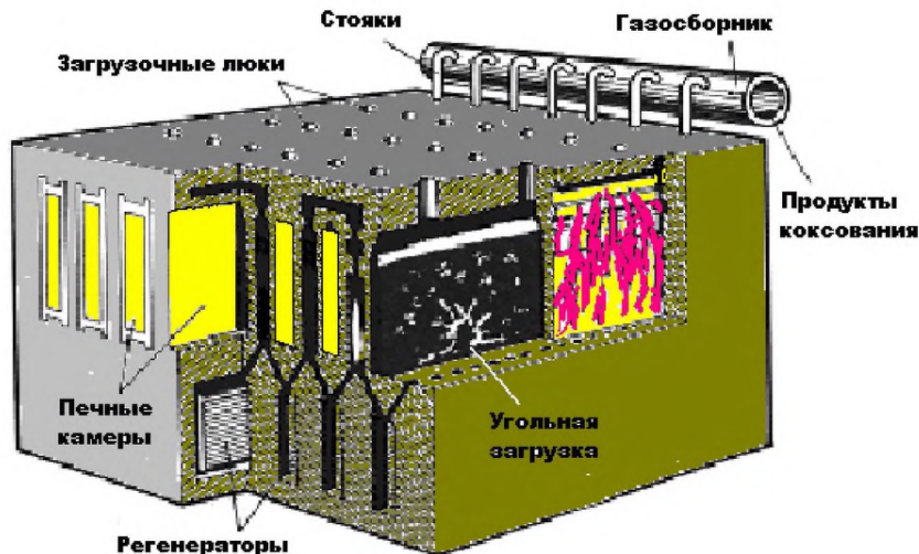
Рисунок 2.19 — Схема устройства коксовой батареи
