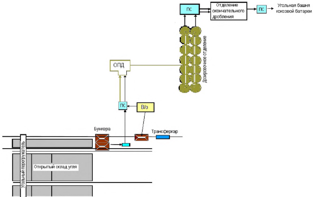
Рисунок 2.18 — Технологическая схема углеподготовки (пример)
