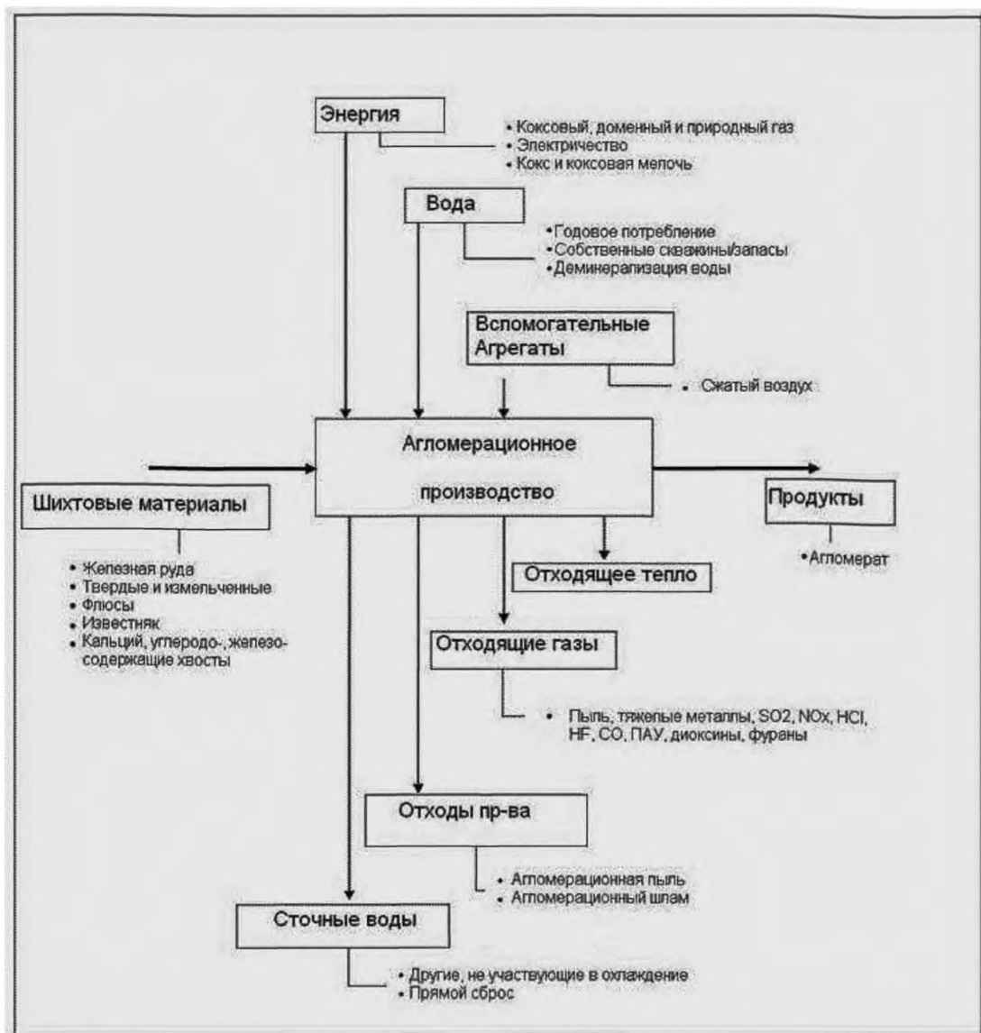
Рисунок 3.2 — Схема материальных потоков на агломерационном производстве [113]
