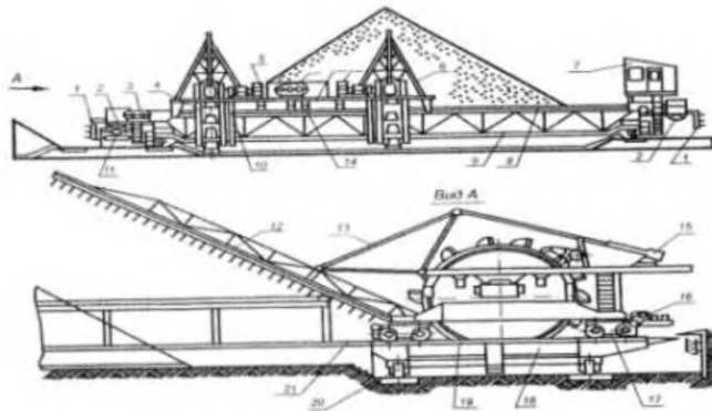
Рисунок 2.7 — Усреднитель роторный У2Р-600
