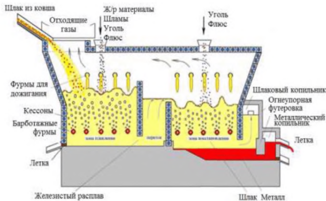
Рисунок 7.16 — Процесс «РОМЕЛТ»
