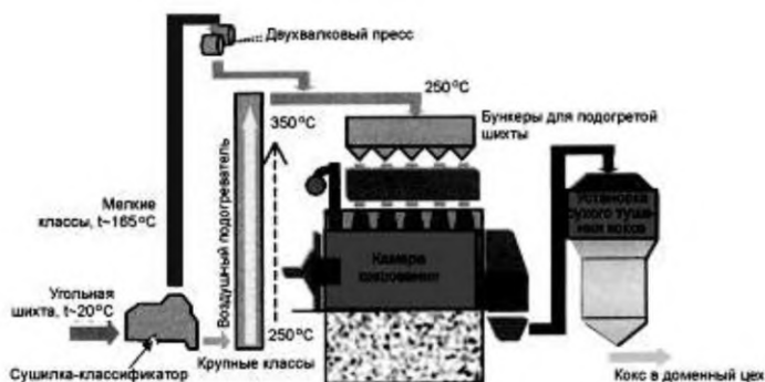
Рисунок 7.7 — Схема технологии частичного брикетирования шихты
