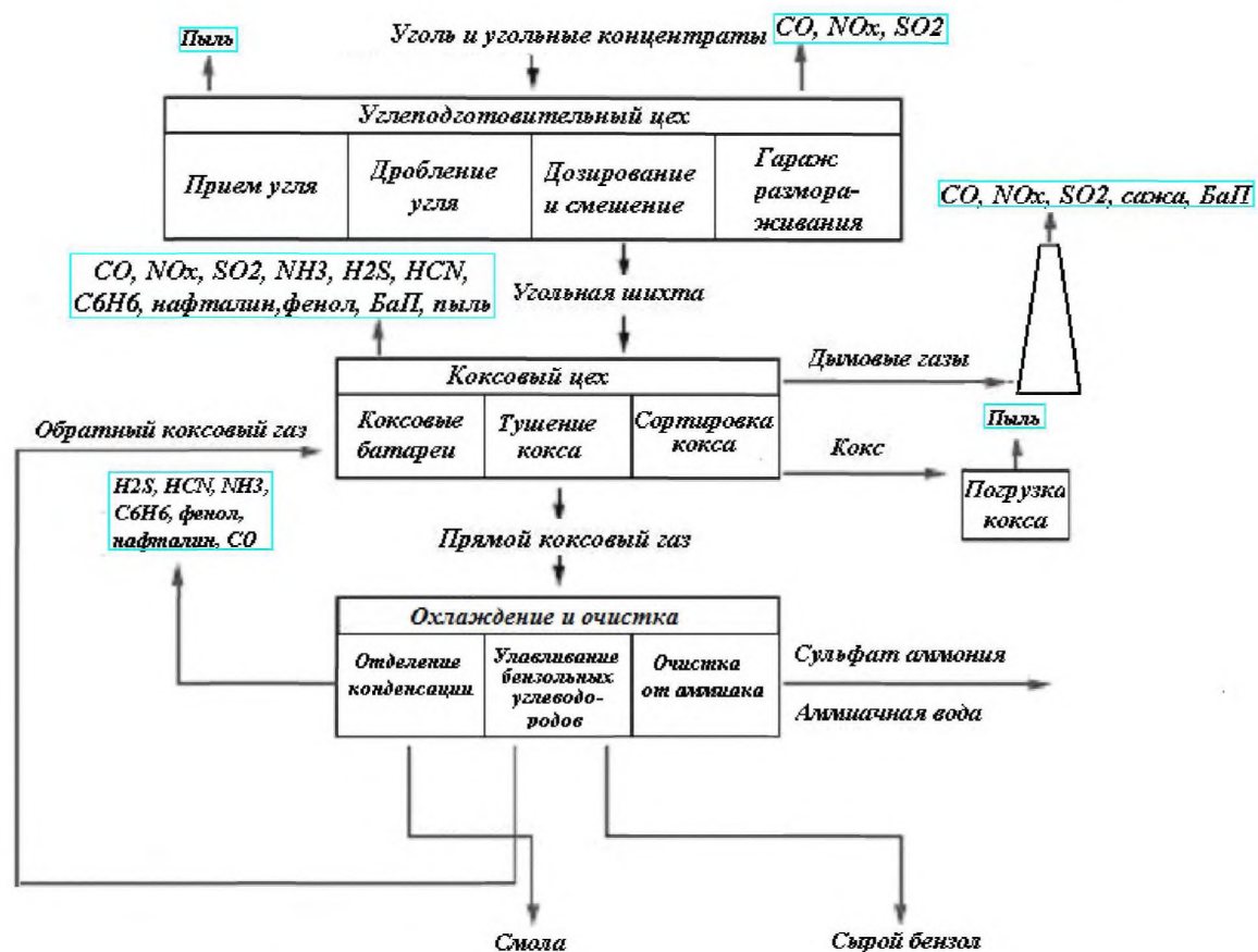
Рисунок 3.4 — Схема формирования выбросов в атмосферу при производстве кокса
