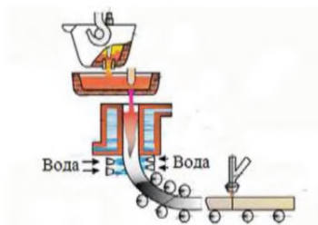
Рисунок 5.8 — Разливка стали на МНЛЗ
