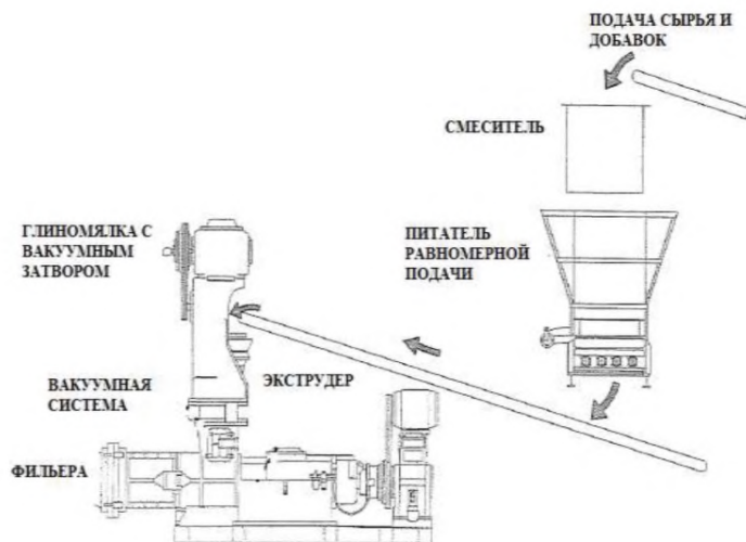
Рисунок 7.4 — Технологическая схема производства брикетов методом жесткой экструзии [165]
