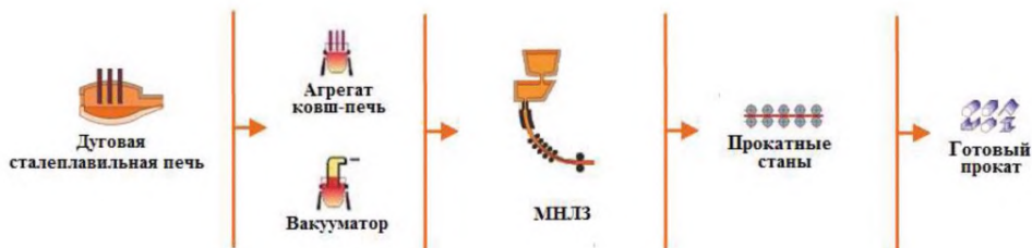
Рисунок 1.5 — Технологическая схема производства «мини-завода» [4]
