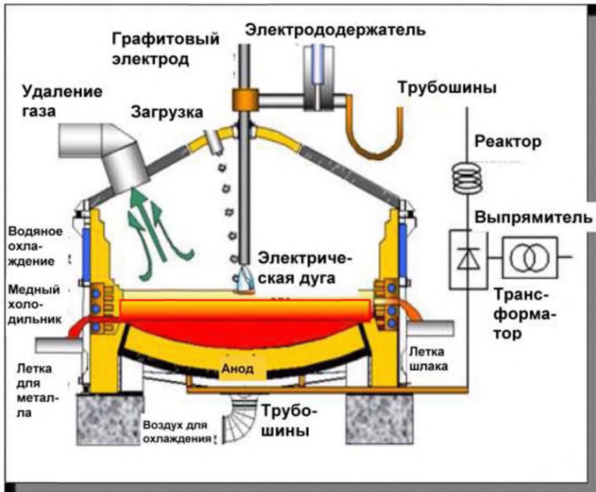
Рисунок 7.26 — Принципиальная схема печи постоянного тока
