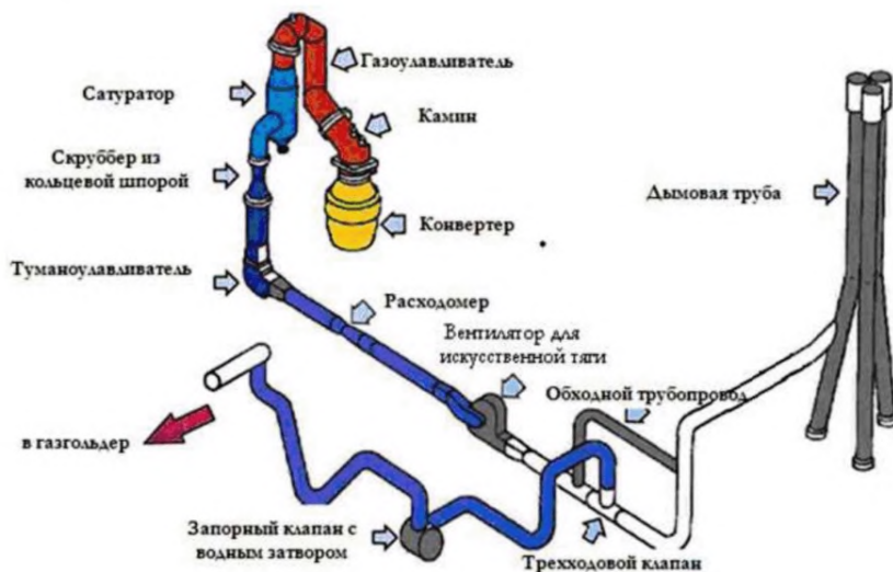
Рисунок 5.9 — Принципиальная схема газоотводящего тракта сталеплавильного конвертера
