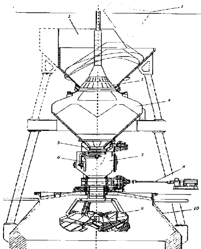
1 — скип; 2 — приемная воронка; 3 — шихтовый и газовый затвор конусного типа; накопительный бункер; 4 — шихтовый клапан; 5 — газовый клапан; 6 — корпус клапанов; 7 — привод ротора; 8 — ротор; 9 — ротор; 10 — купол печи
