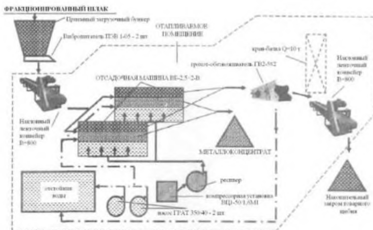
Рисунок 2.74 — Технологическая схема гравитационного обогащения шлака высокоуглеродистого феррохрома
