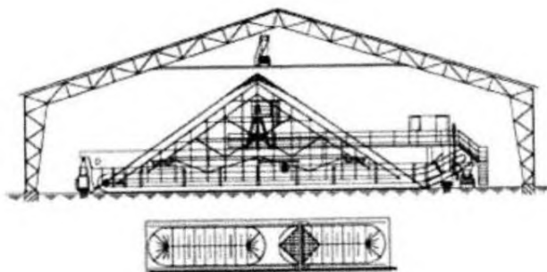
Рисунок 2.8 — Закрытый усреднительный склад
