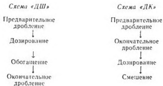
Рисунок 2.17 — Схемы подготовки углей к коксованию
