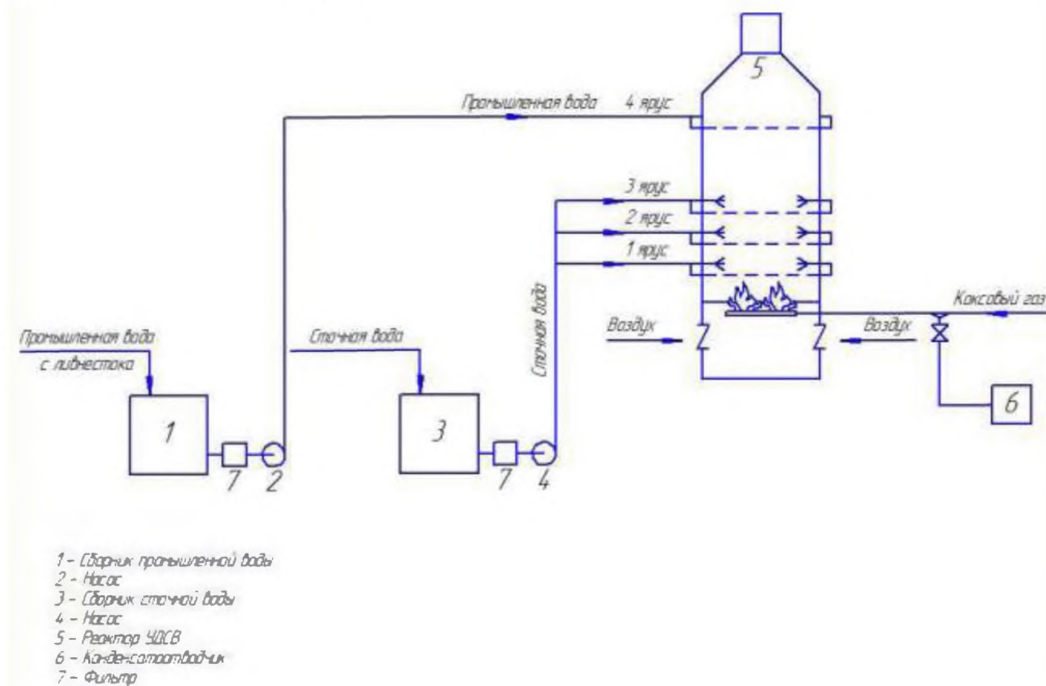
Рисунок 7.12 — Схема установки сжигания сточных вод
