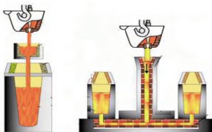
слева — наполнение изложницы сверху; справа — наполнение изложницы с помощью сифона
