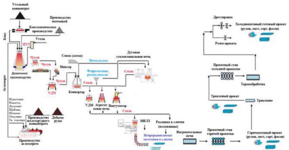
Рисунок 1.4 — Схема производства металлопродукции на интегрированном предприятии
