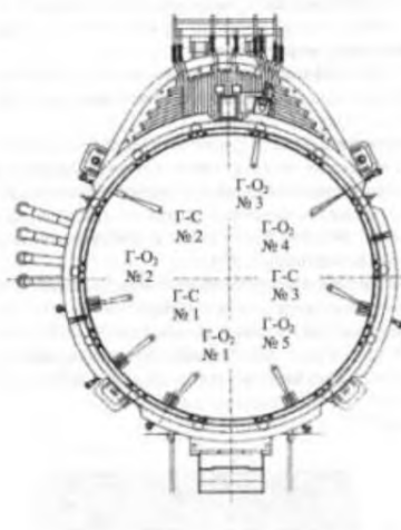
Рисунок 2.50 — Типичное расположение инжекторов в ДСП
