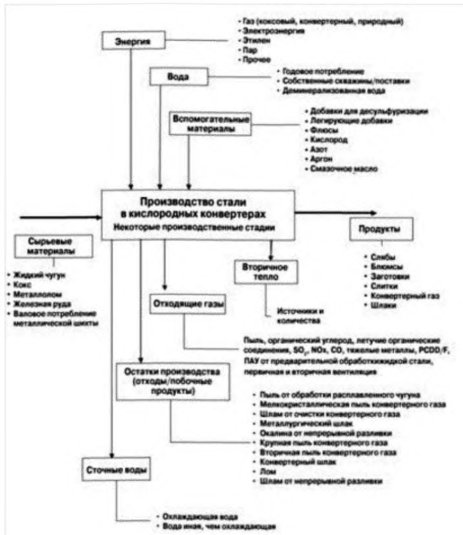
Рисунок 3.13 — Схема материальных потоков при кислородно-конвертерном производстве стали [113]
