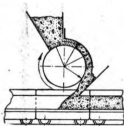
Рисунок 2.9 — Барабанный питатель с наклонным загрузочным лотком
