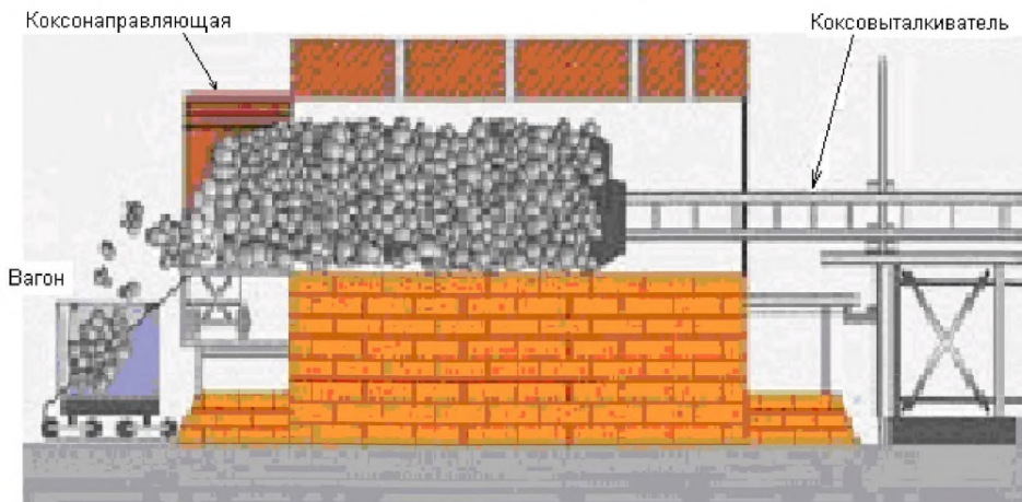
Рисунок 2.20 — Схема выдачи кокса
