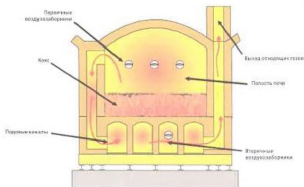
Рисунок 7.11 — Разрез печи рекуперативного типа
