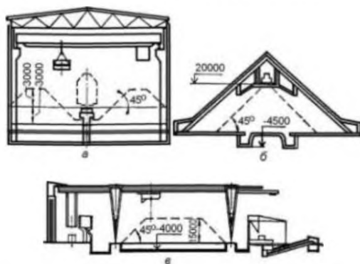
а — закрытый грейферный; б — закрытый бескрановый; в — открытый
