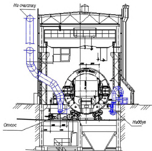
Рисунок 7.6 — Схема аспирации вагонопрокидывателя
