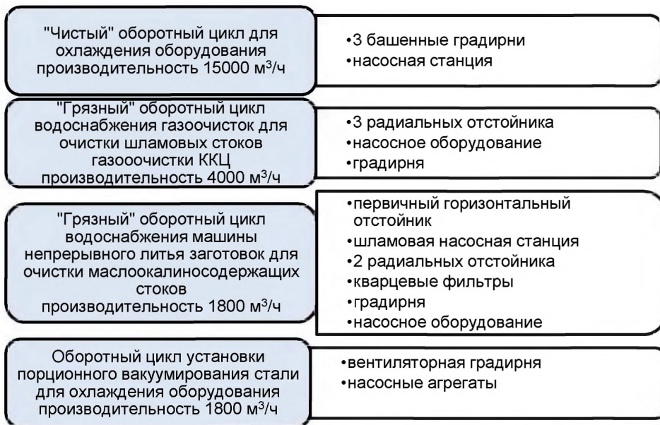
Рисунок 3.15— Оборотная схема водоснабжения кислородно-конвертерного цеха ПАО «ММК» [122]
