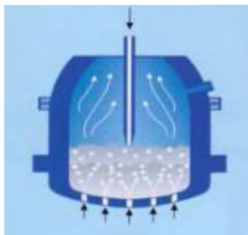
Рисунок 5.5 — Комбинированная продувка в конвертере (сверху и донная)
