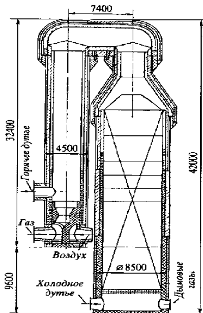
Рисунок 2.32 — Воздухонагреватель с выносной камерой горения
