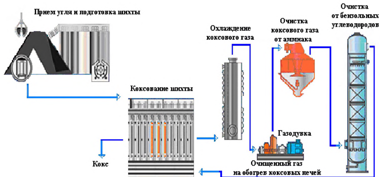
Рисунок 2.16 — Принципиальная схема производства кокса
