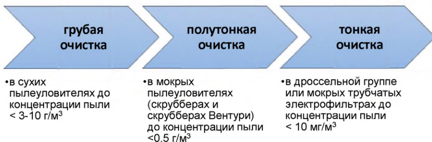
Рисунок 3.10 — Многоступенчатая система очистки доменного газа
