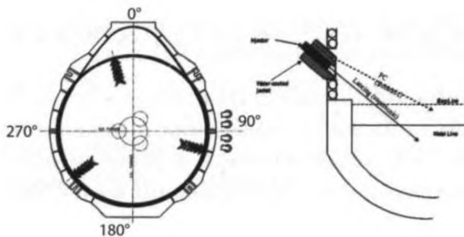
Рисунок 2.50 — Типичное расположение инжекторов в ДСП
