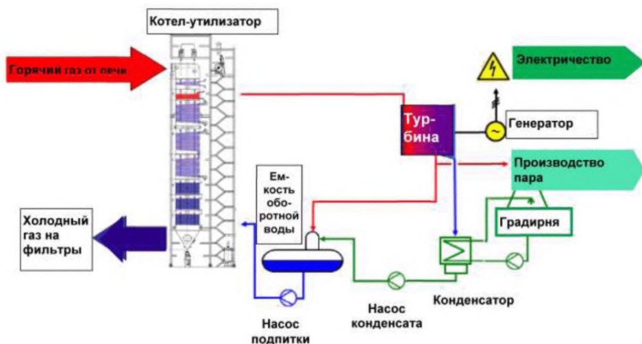
Рисунок 7.25 — Типичная блок-схема рекуперации энергии при выплавке ферросплава
