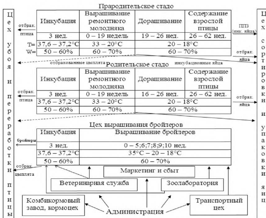
Рис. 2.2 – Схема технологического процесса производства бройлеров
