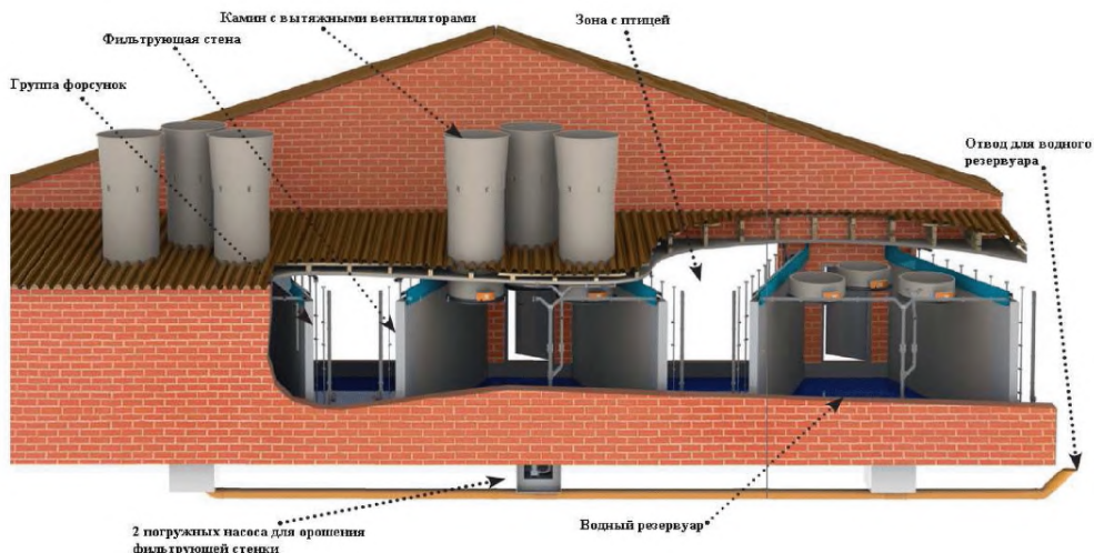
Рис. 7.2 — Схематическое изображение очистителя воздуха
