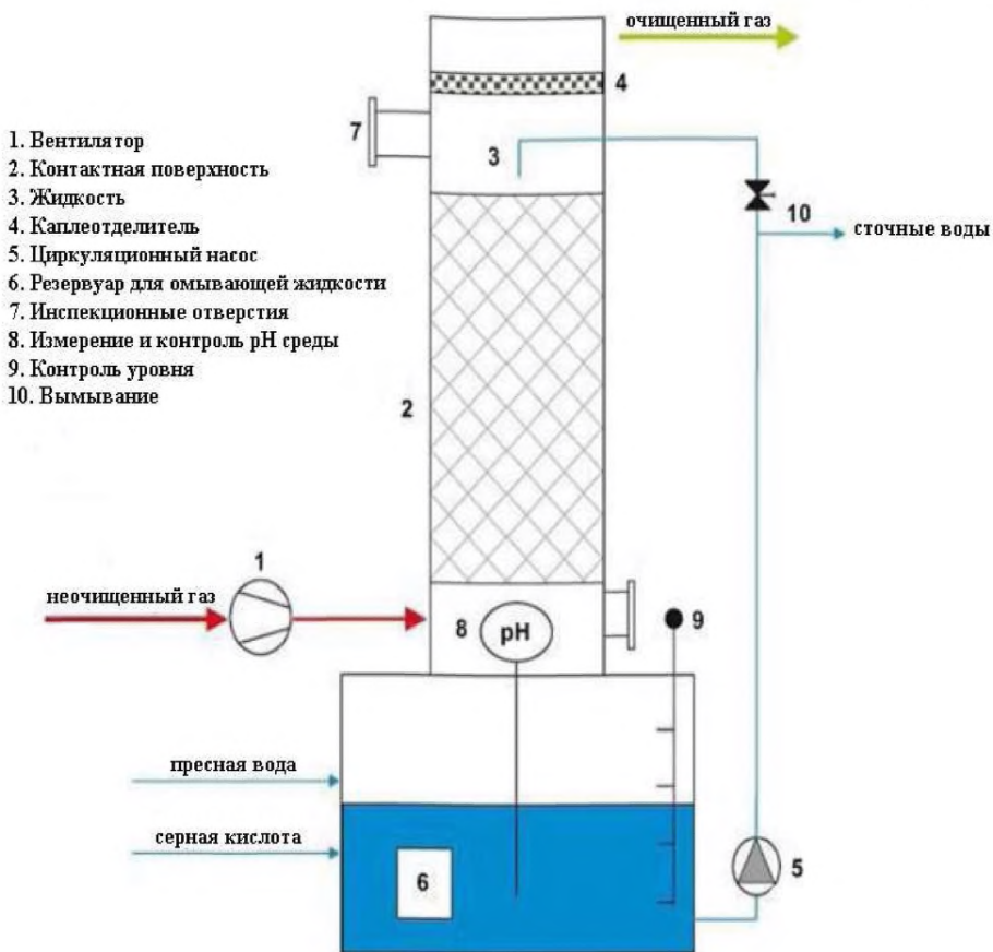
Рис. 7.1 — Рабочий процесс биоскруббера
