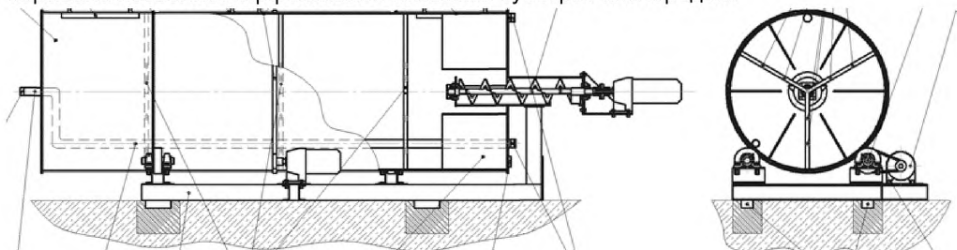
Рисунок 2.13 — Общая схема биоферментатора барабанного типа
