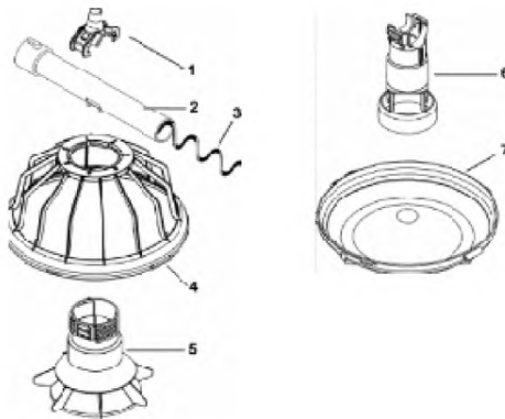
Рис. 2.5 – Основные элементы кормушек тарелочного типа:
