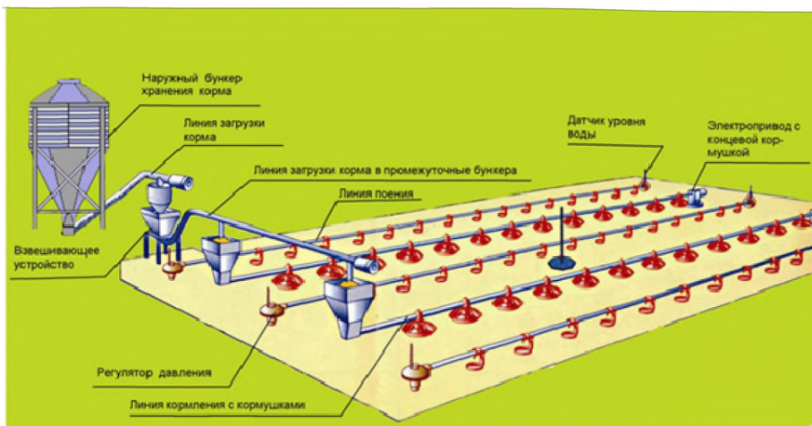
Рисунок 2.8 — Оборудование для напольного выращивания бройлеров
