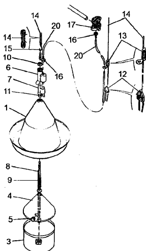
Рисунок 2.6 — Круглая поилка: 1 – колокол поилки; 3 – нижняя часть поилки; 4 – крышка; 5 – заглушка; 6 – корпус клапана внешний; 7 – корпус клапана внутренний; 8 – подвесной стержень; 9 – пружина большая; 10 – контргайка; 11 – клапанное устройство; 12 – натяжное устройство для подвесного каната; 13 – направляющие шланги; 14 – подвесной канат; 15 – S-крюк; 16 – наконечник; 17 – заслонка; 20 – шланг
