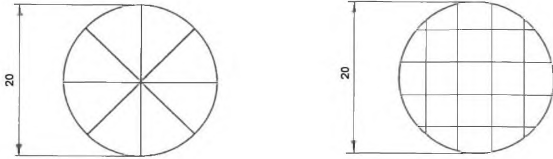
Рисунок 12 – Образец царпин для испытаний на взрывоопасность
