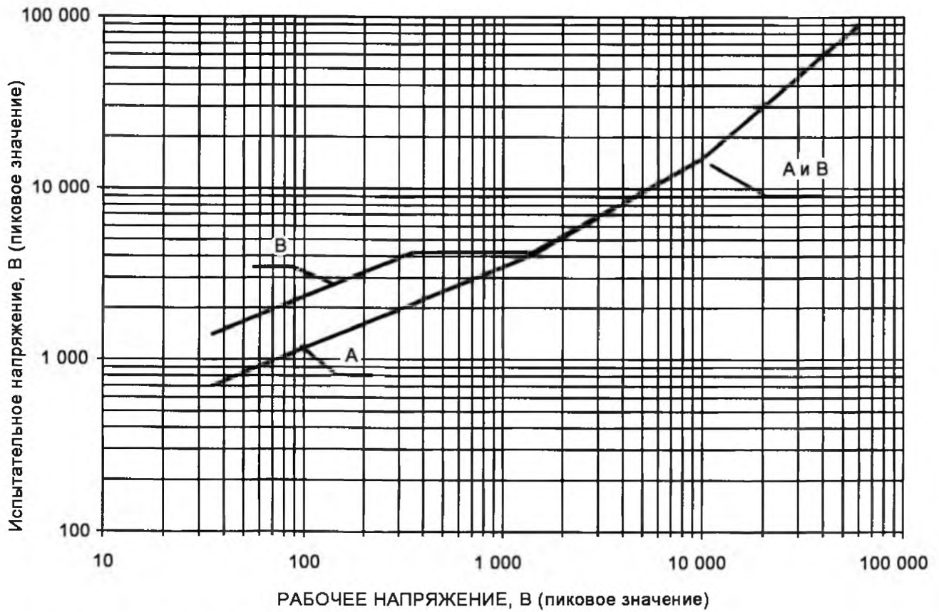
Рисунок 7 – Испытательное напряжение
