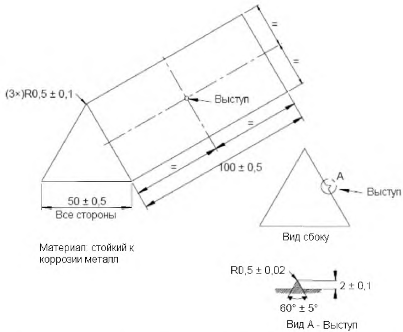
Рисунок 14 – Оправка
