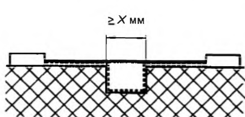
Рисунок Е.1 – Узкая канавка
