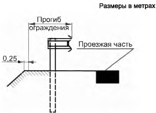
Рисунок Г.2 – Расположение деформируемого дорожного ограждения на обочине
