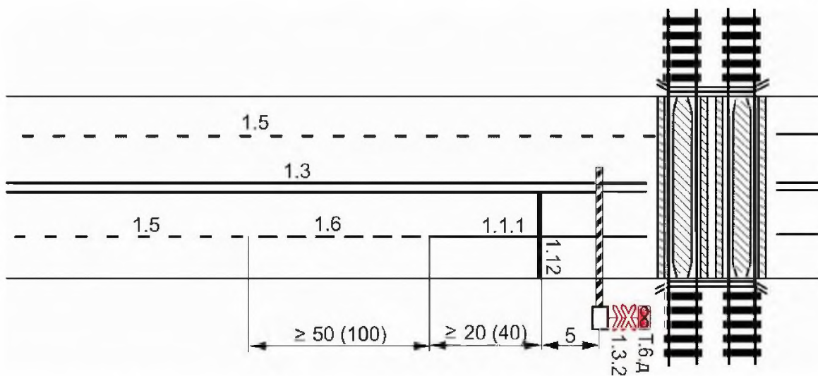
Рисунок В.11 – Нанесение разметки перед железнодорожным переездом со шлагбаумом
