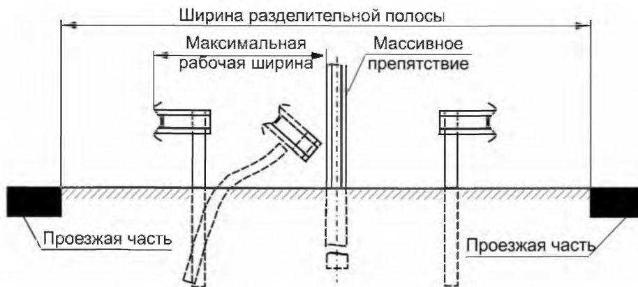
Рисунок Г.4 – Рабочая ширина дорожного ограждения, установленного на разделительной полосе
