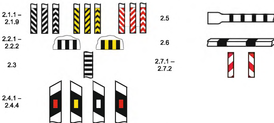
Рисунок Б.2 – Вертикальная дорожная разметка
