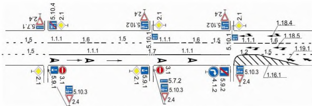
Рисунок В.9 – Выделение разметкой полос для встречного движения маршрутных транспортных средств
