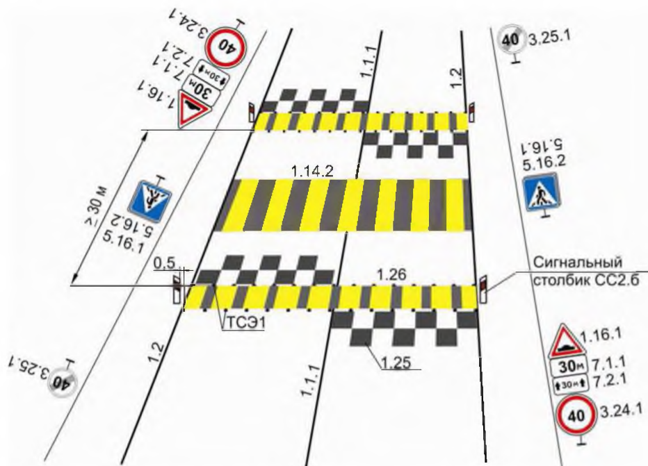
Рисунок Л.3 – Пример обозначения искусственной неровности ИН 1
