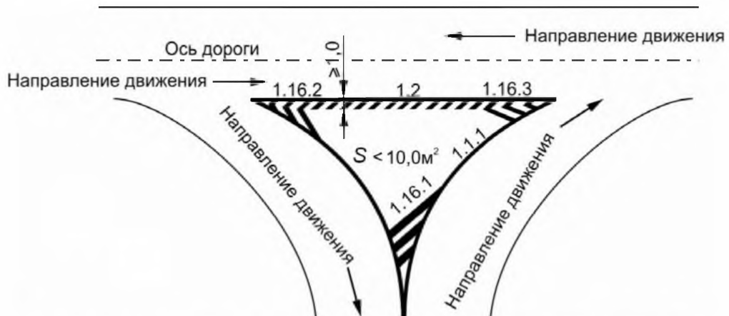
Рисунок В.20 – Нанесение разметки при обозначении направляющих островков
