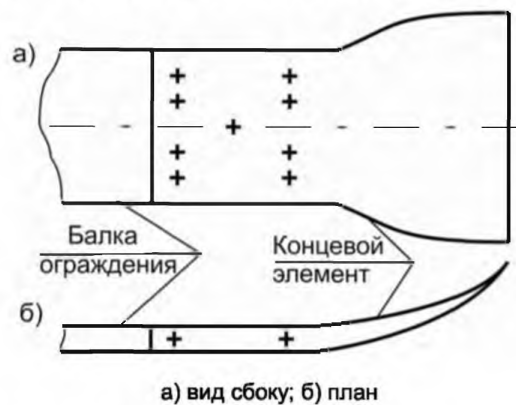
Рисунок Г.8 – Конструкция концевой элемент начального участка дорожного ограждения
