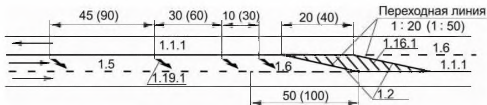
Рисунок В.8 – Нанесение разметки при уменьшении полос движения в данном направлении
