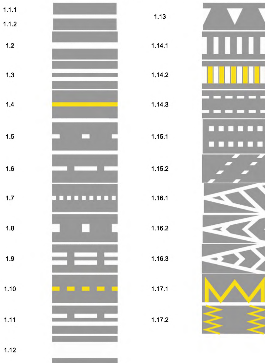
Рисунок Б.1, лист 1 – Горизонтальная дорожная разметка
