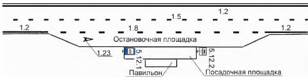
Рисунок В.17 – Нанесение разметки на остановочных площадках маршрутных транспортных средств
