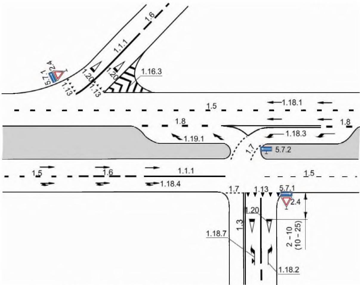
Рисунок В.19 – Обустройство перекрестков со сложной планировкой
