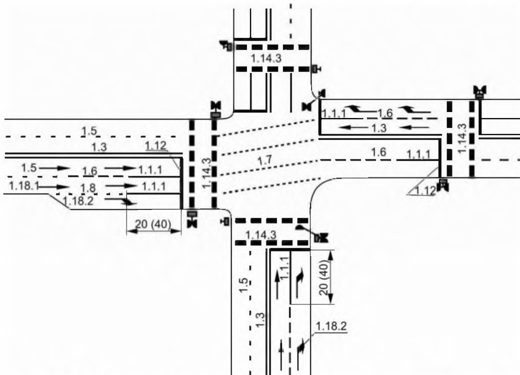
Рисунок В.10 – Нанесение разметки перед регулируемыми пешеходными переходами
