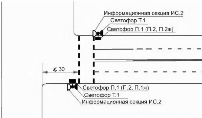
Рисунок К.5 – Установка информационной секции ИС.2
