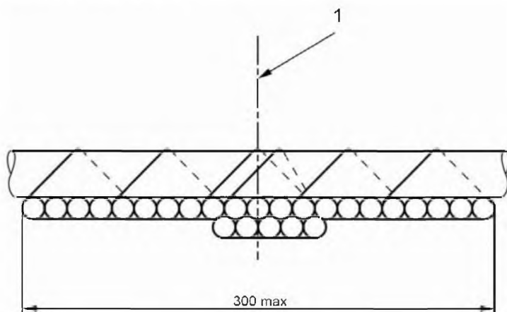
Рисунок 3 – Отрезки кабеля, закрепленные без зазора на передней стороне стандартной лестницы (совокупности отрезков кабеля находятся в непосредственном контакте)
