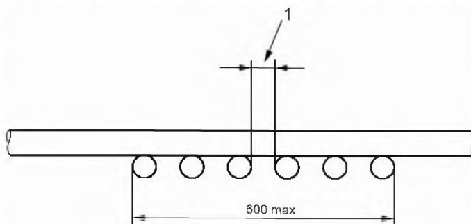
Рисунок 1 – Отрезки кабеля, закрепленные с зазором на передней стороне стандартной лестницы
