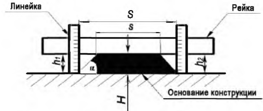
Рисунок 8.2 – Схема измерения искусственной неровности трапецевидной формы
