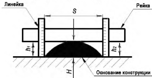
Рисунок 8.1 – Схема измерения искусственной неровности криволинейной формы
