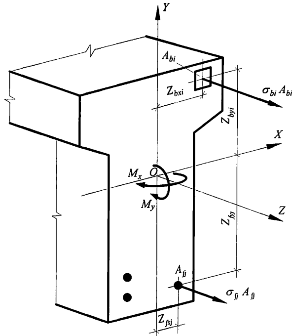
Рисунок 5 – Расчетная схема нормального сечения конструкции
