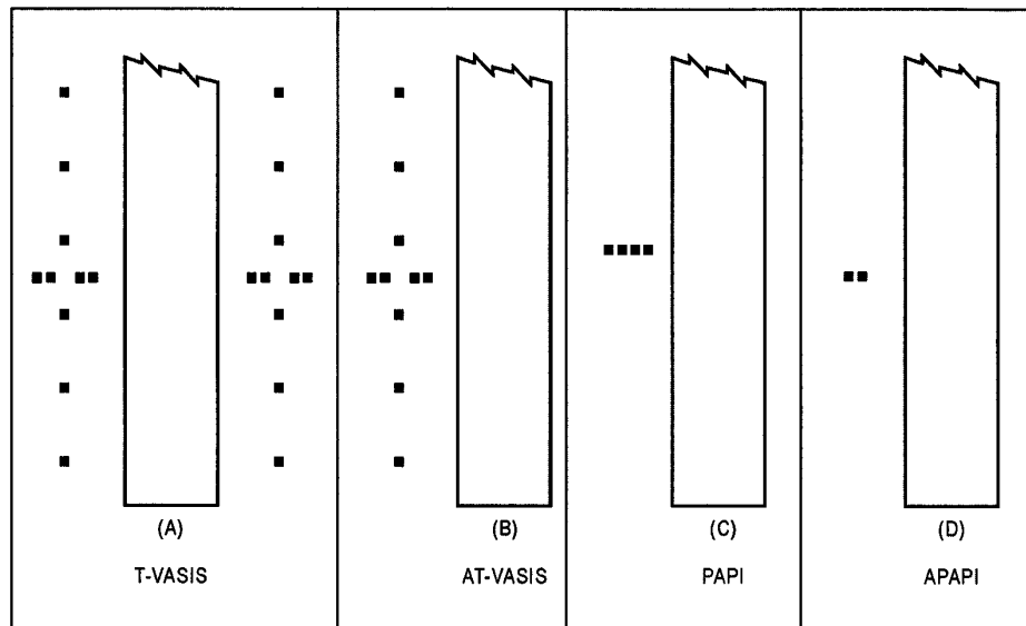
Рис. 5-16. Системы визуальной индикации глиссады
