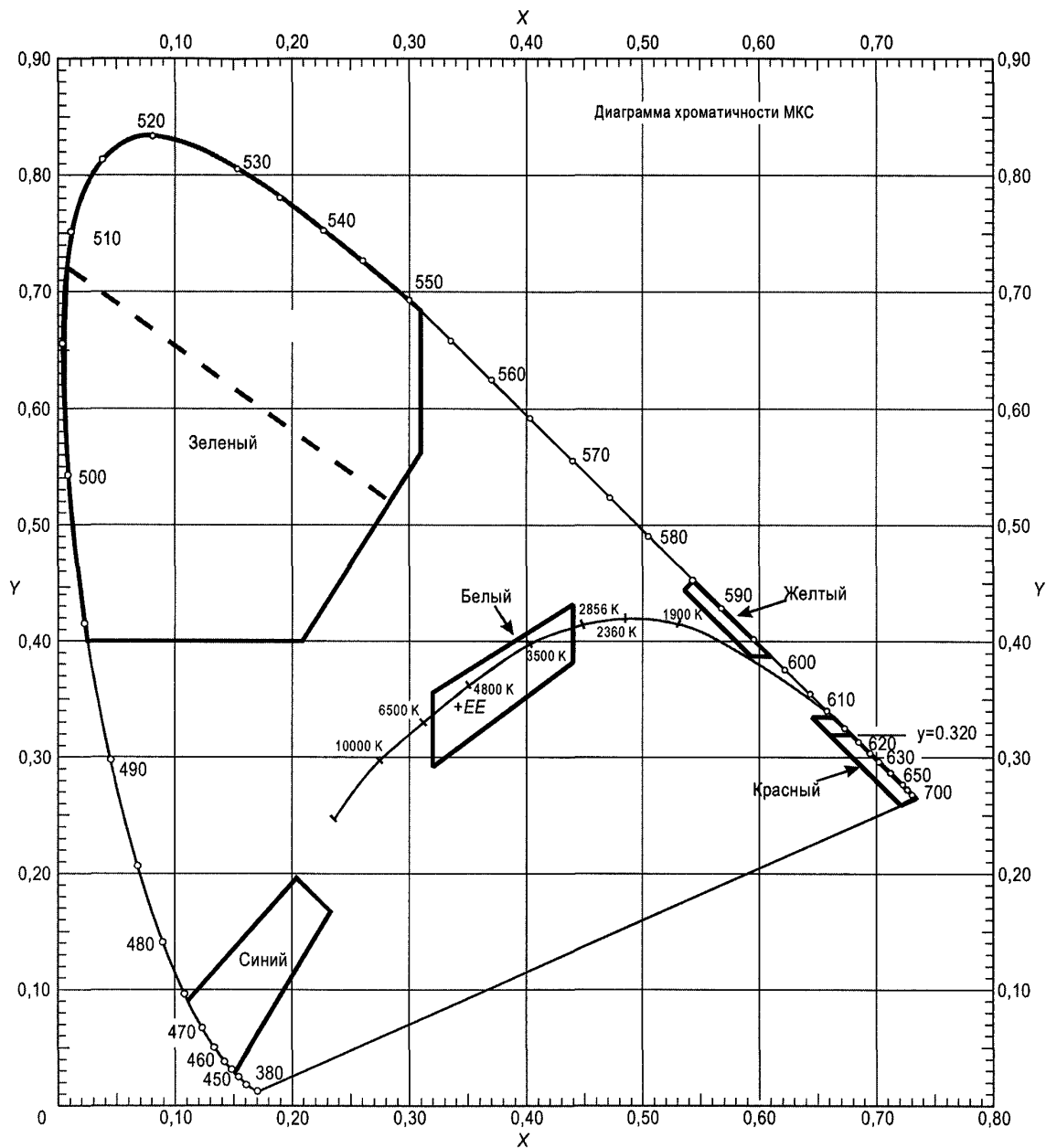
Рис. А1-1в. Цвета аэронавигационных наземных огней (твердотельные источники света)
