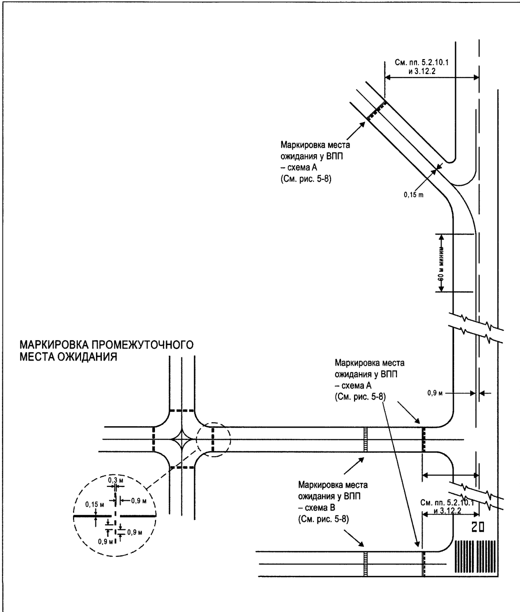
Рис. 5-6. Маркировка РД (указано вместе с основной маркировкой ВПП)
