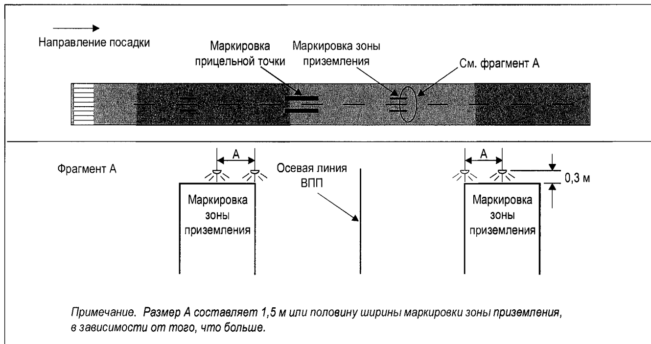
Рис. 5-24. Простые огни зоны приземления
