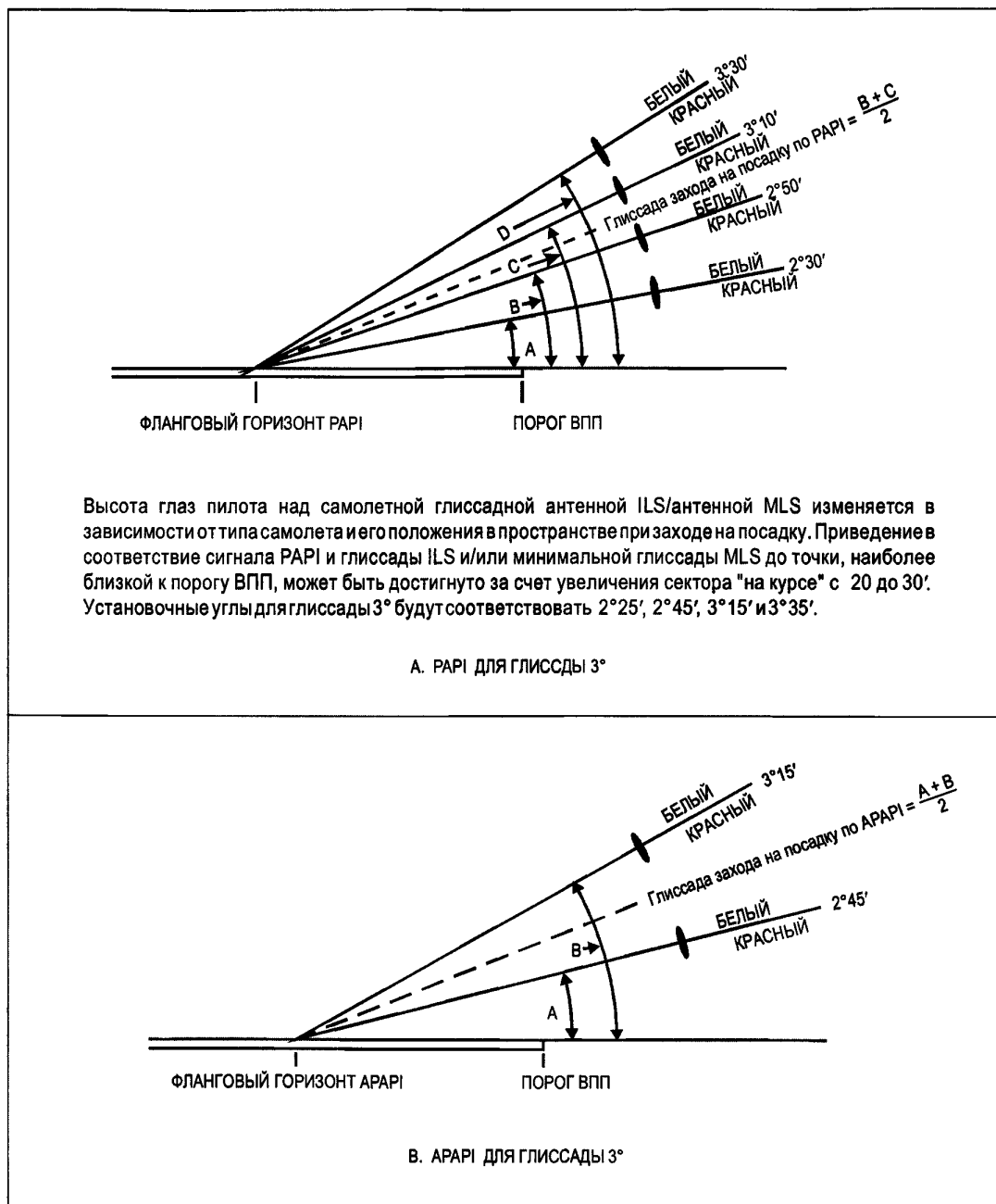
Рис. 5-20. Световые лучи и установка углов возвышения РАРІ и АРАРІ
