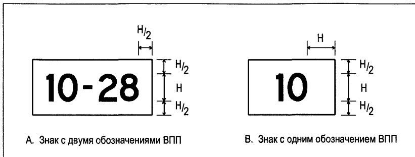
Рис. А4-4. Размеры знака
