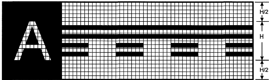
Знак освобожденной ВПП (с типовым знаком местоположения)
