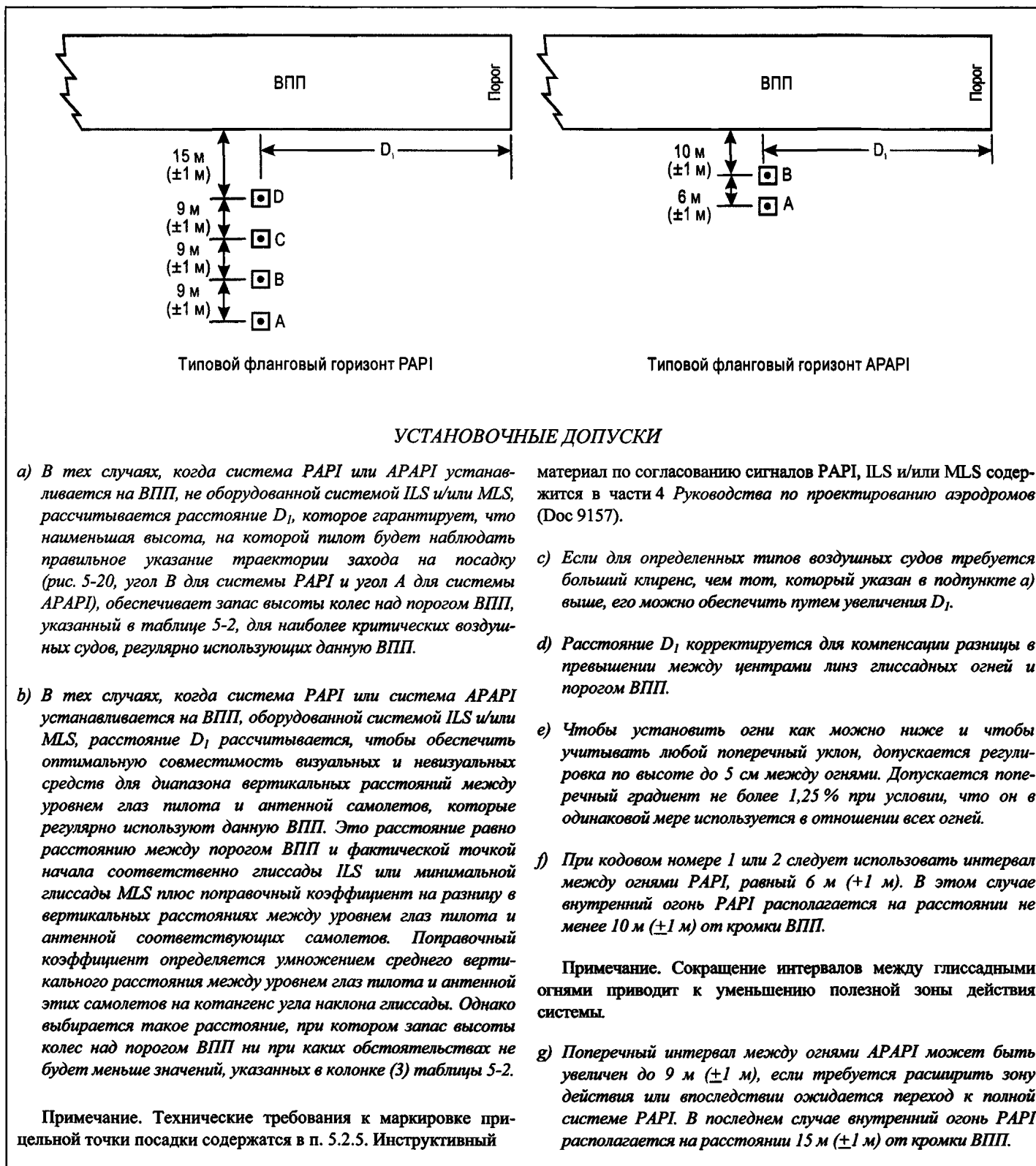
Рис. 5-19. Расположение PAPI и APAPI
