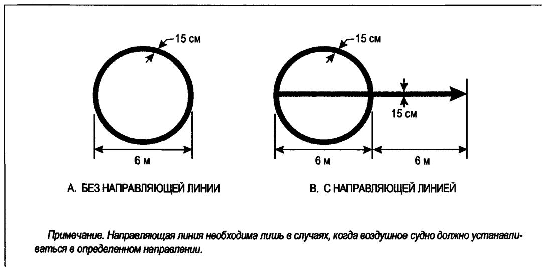
Рис. 5-9. Маркировка аэродромного пункта проверки VOR
