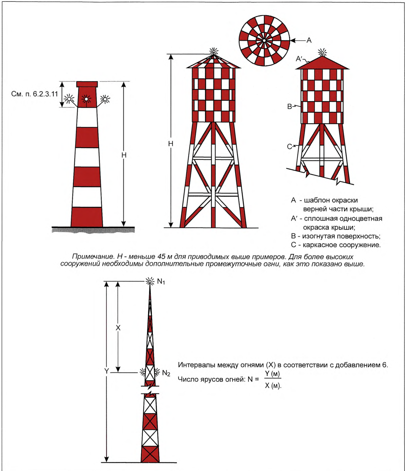
Рис. 6-2. Примеры маркировки и светового ограждения высоких сооружений
