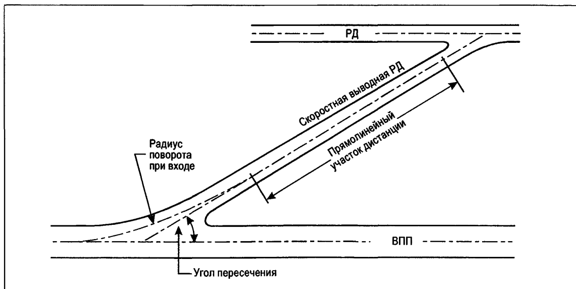
Рис. 3-3. Скоростная выводная РД
