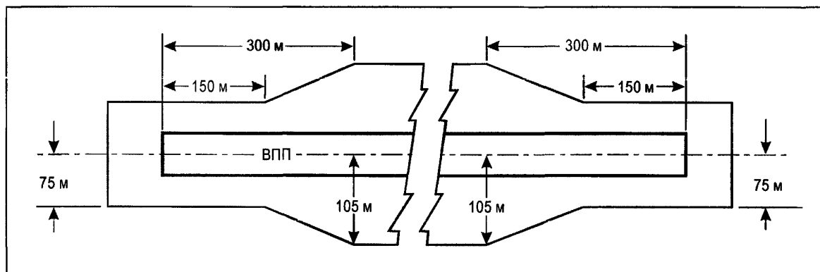
Рис. А-4. Спланированный участок полосы, включающий ВПП, оборудованную для точного захода на посадку, с кодovým обозначением 3 или 4
