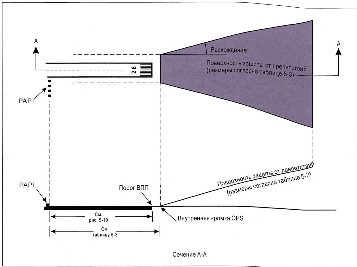
Рис. 5-21. Поверхность защиты от препятствий для систем визуальной индикации глассдады
