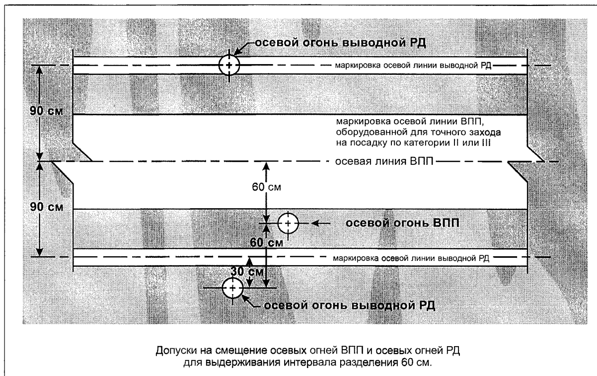
Рис. 5-27. Смещенные осевые огни ВПП и РД
