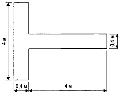
Рис. 5-1. Указатель направления посадки
