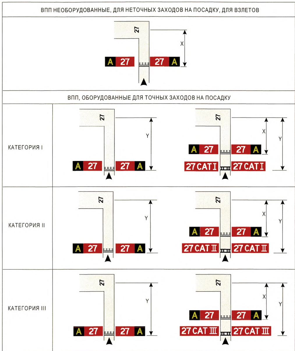
Рис. 5-32. Примеры расположения знаков на пересечениях РД/ВПП
