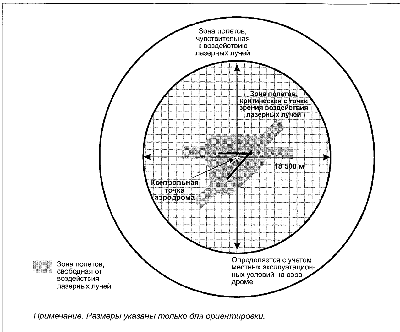
Рис. 5-11. Защищенные зоны полетов
