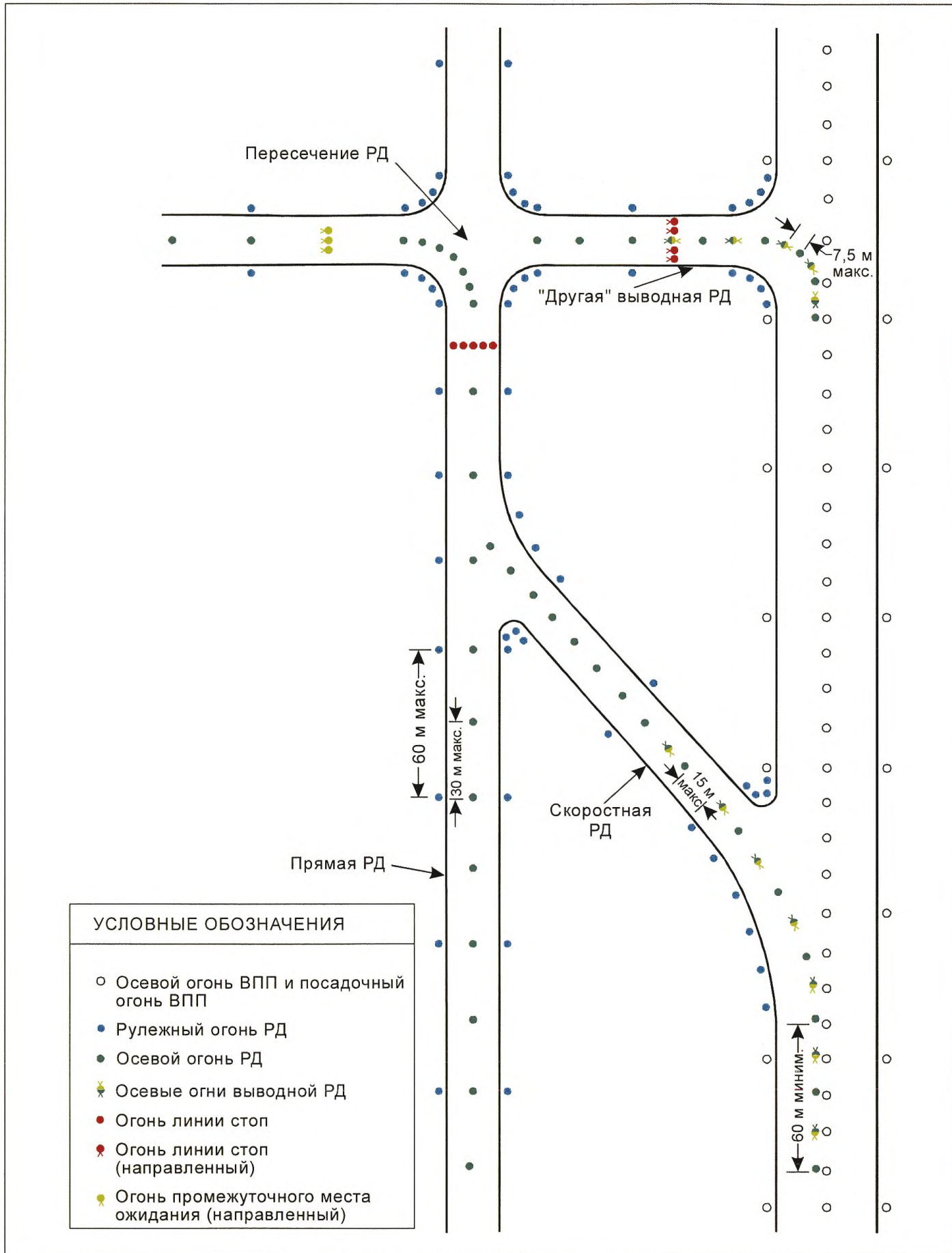
Рис. 5-26. Светосигнальная система РД
