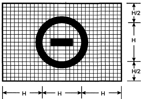
Знак "ВЪЕЗД ЗАПРЕЩЕН"
