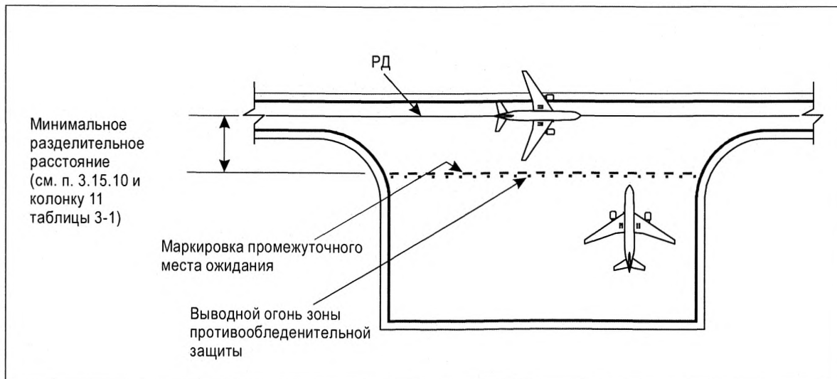
Рис. 5-28. Типичная удаленная зона противообледенительной защиты
