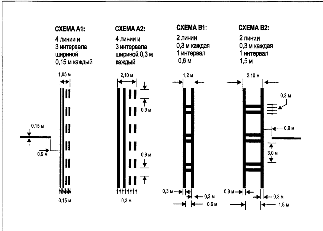
Рис. 5-8. Маркировка места ожидания у ВПП Примечание. После 2026 года схемы А1 и В1 применяться не будут.
