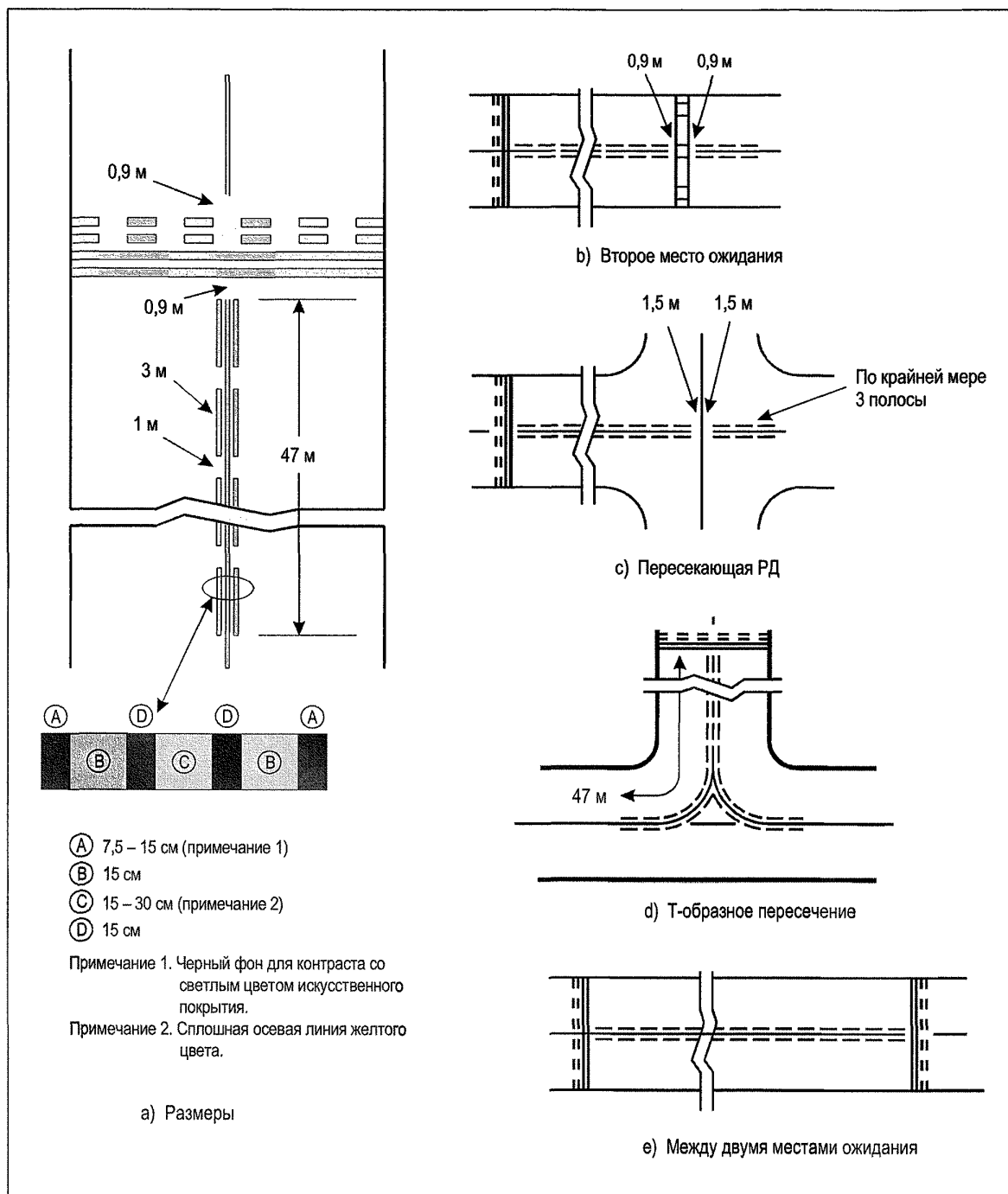
Рис. 5-7. Улучшенная маркировка осевой линии РД
