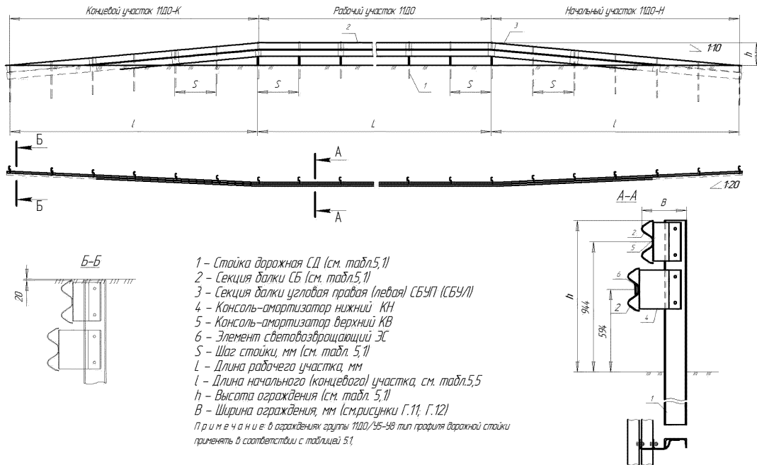
Рисунок Г.3 – Ограждение группы 11Д0/У5-У8
