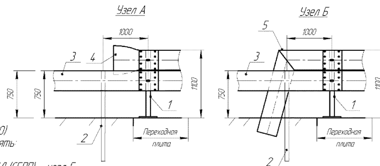
Рисунок Г.23 – Сопряжение дорожной группы 11ДО/У5-У9 с мостовой группой 11МО/У4-У10
