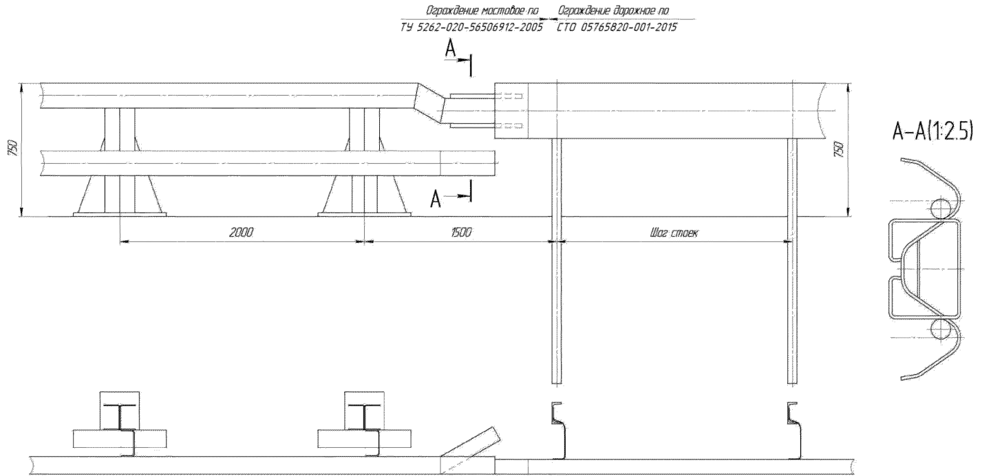
Рисунок Д.15 – Узел сопряжения мостового ограждения (ТУ 5262-020-56506912-2005) с дорожным ограждением
