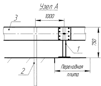
Рисунок Г.22 – Сопряжение дорожной группы 11ДО/У1-У4 с мостовой группой 11МО/У1-У3
