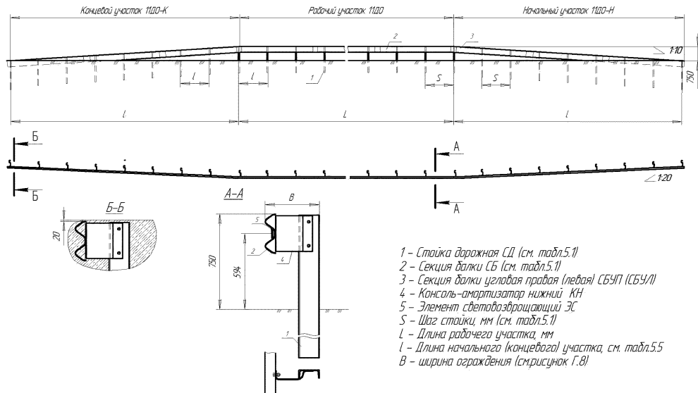
Рисунок Г.1 – Ограждение группы НДО/У1-У4
