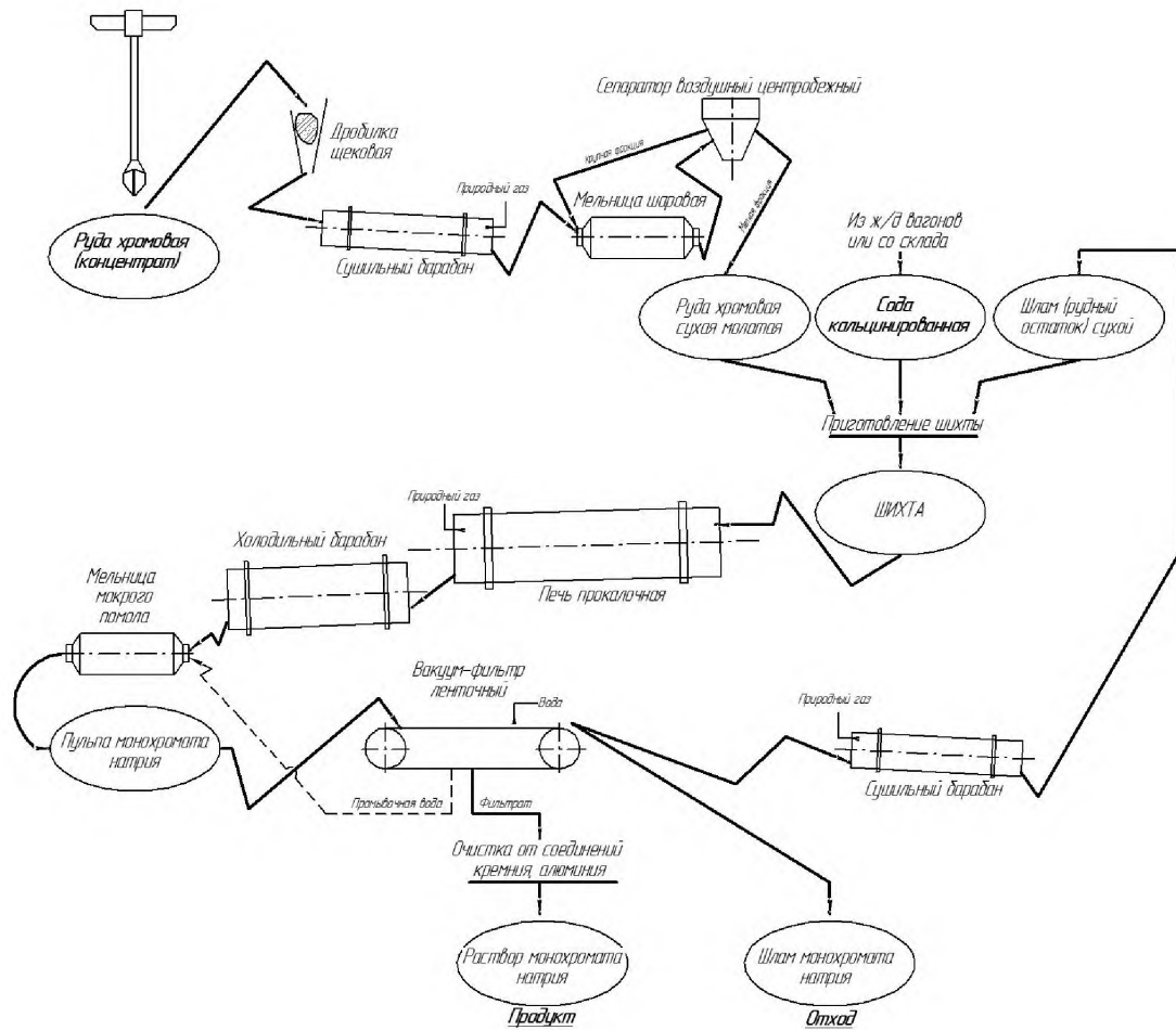
Рисунок 8.2 – Принципиальная схема получения раствора монохромата натрия (бездоломитовый метод)
