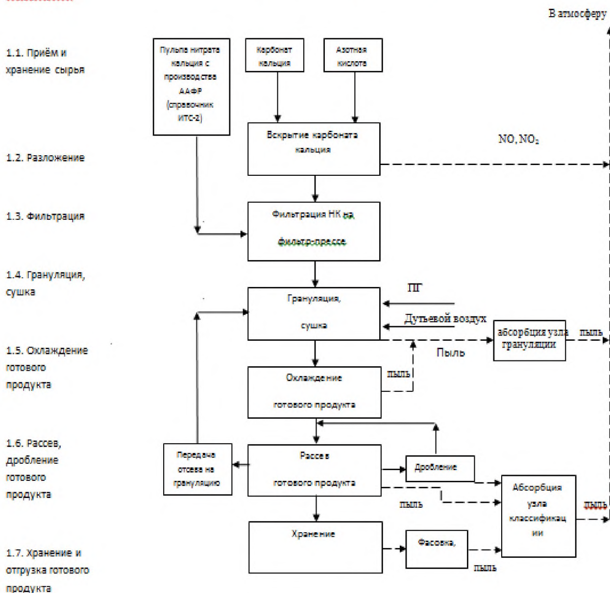
Рисунок 5.2 – Процесс производства гранулированного нитрата кальция
