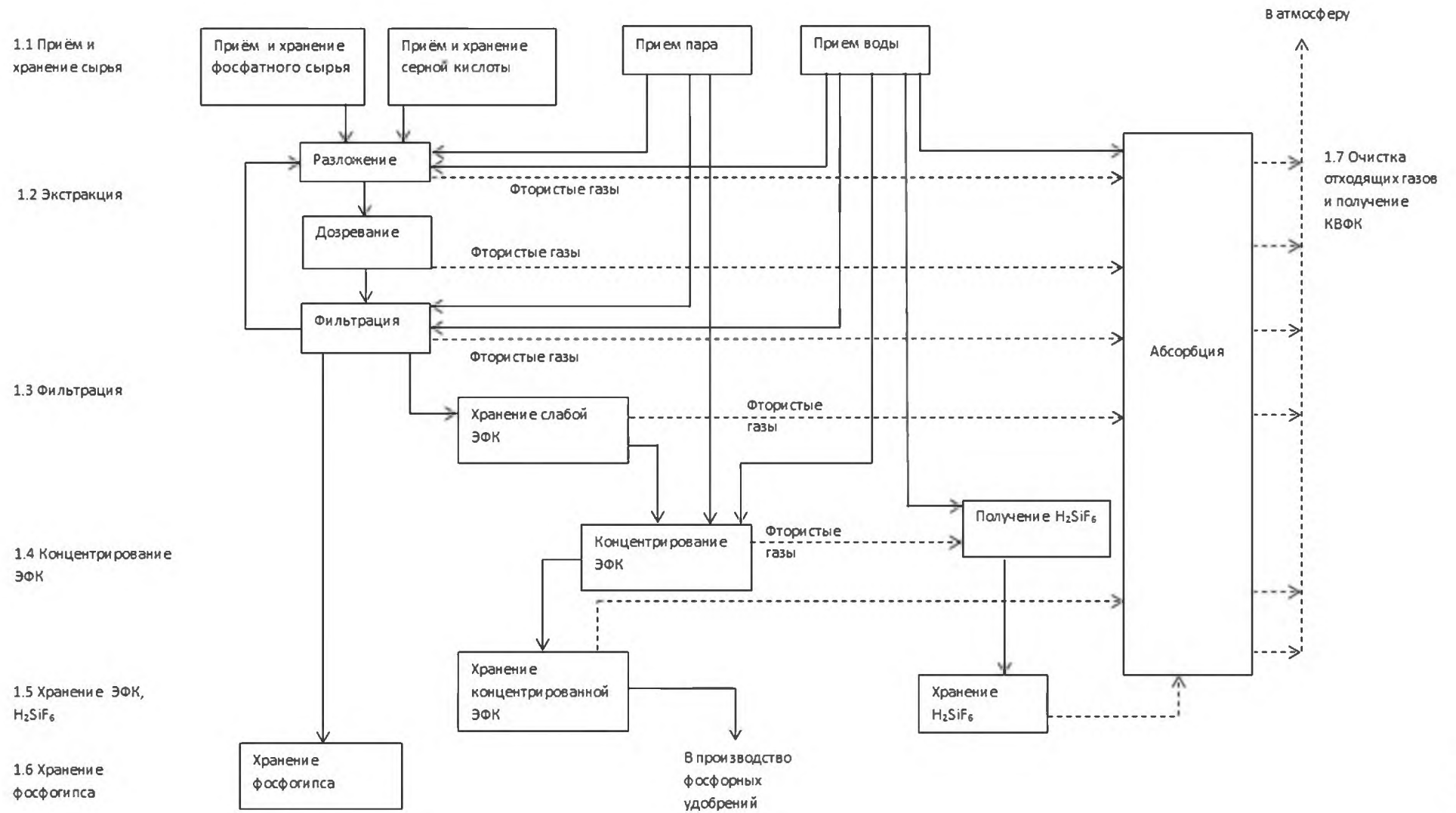
Рисунок 3.2 – Схема получения ЭФК и фосфогипса
