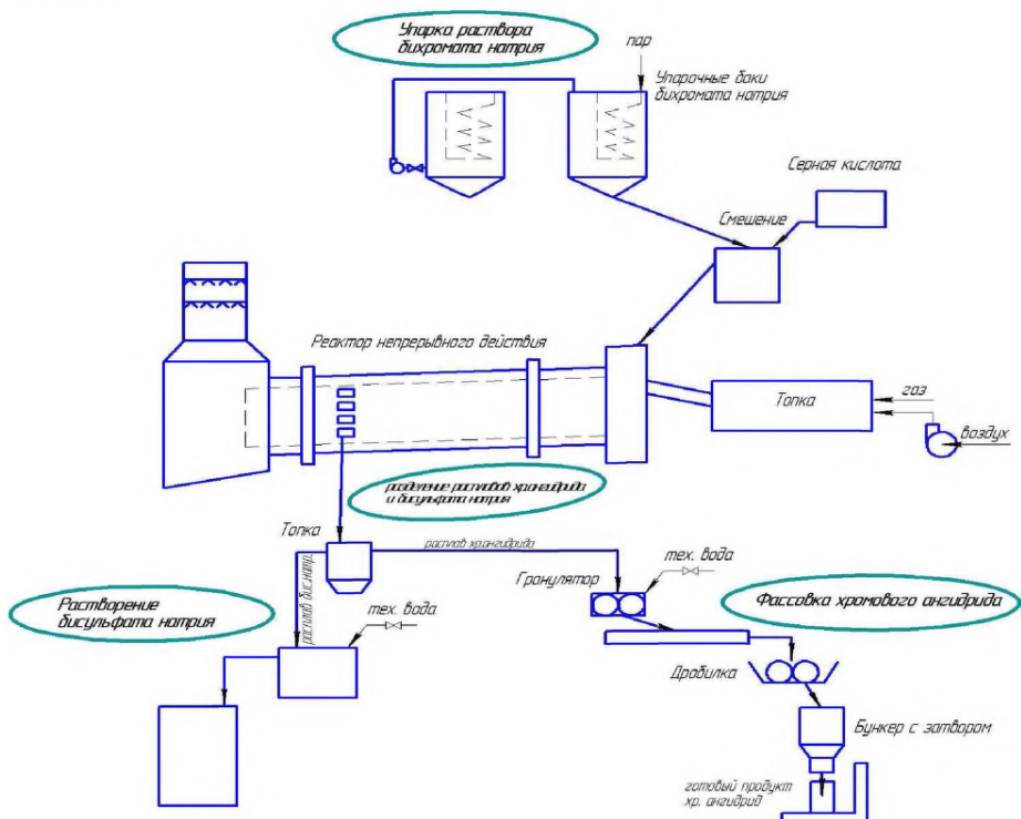
Рисунок 8.4 – Принципиальная схема производства хромового ангидрида
