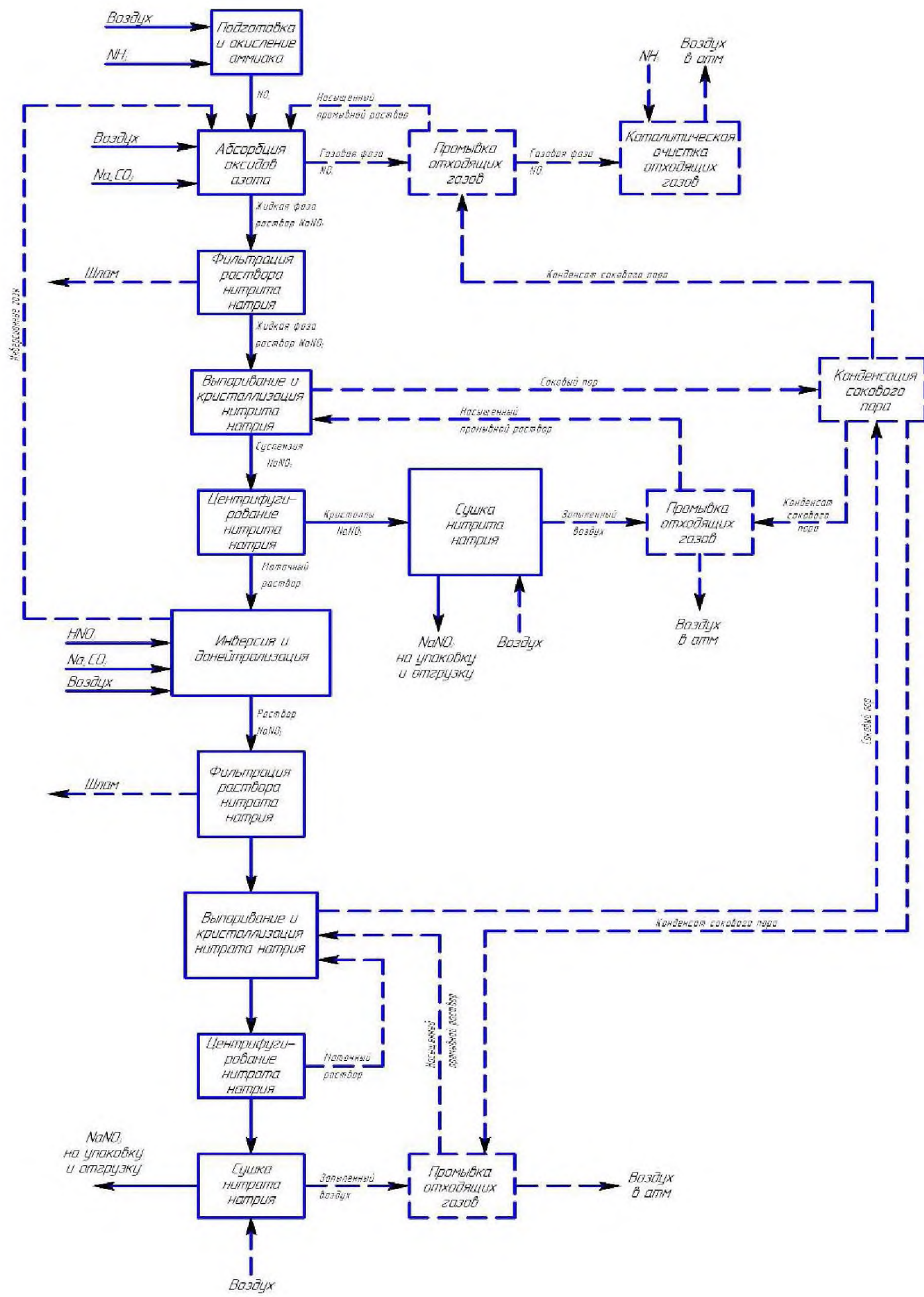
Рисунок 10.2 – Принципиальная схема производства натриевой селитры
