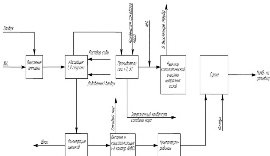
Рисунок 10.1. – Принципиальная схема производства нитрата натрия
